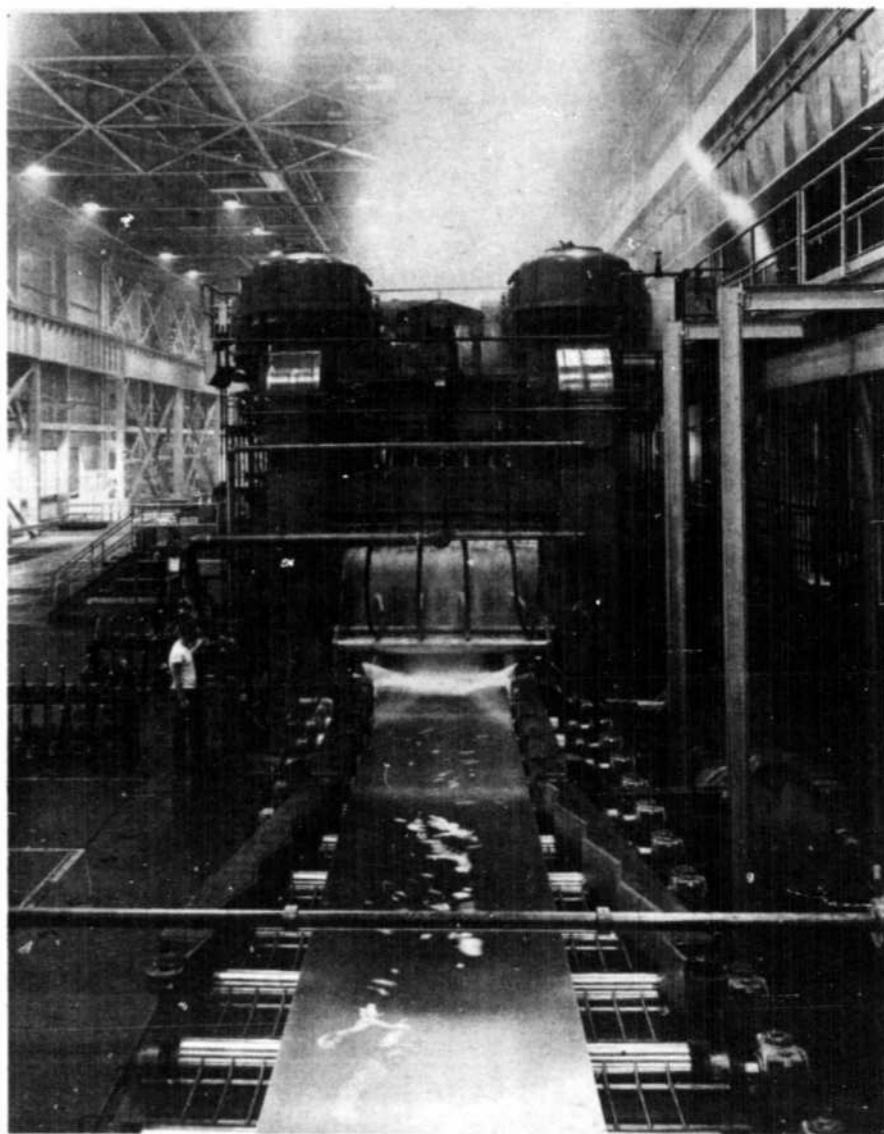
UNE PRESSE du laminoir d'Alroll, à Oswégo, dans l'Etat de New-York. En douze phases successives, un lingot d'aluminium de 18 pouces d'épaisseur est réduit à un pouce. C'est une autre preuve de la présence d'Aluminium Limited au cœur des marchés de ses concurrents.
