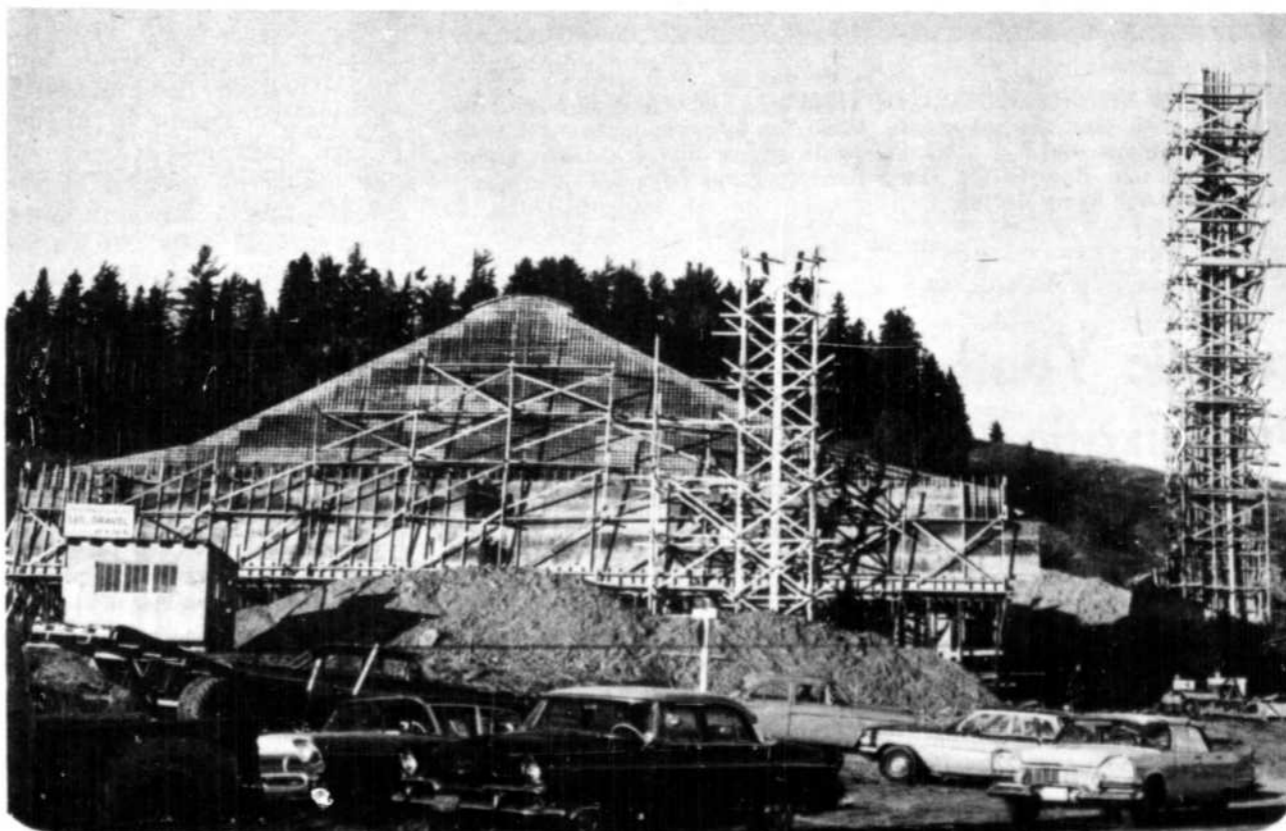
L'ÉGLISE ST-LUC emprunte la forme d'une tente. L'architecte Jacques Coutu tire grand profit du fait qu'il est possible de donner au béton la forme que l'on veut.
