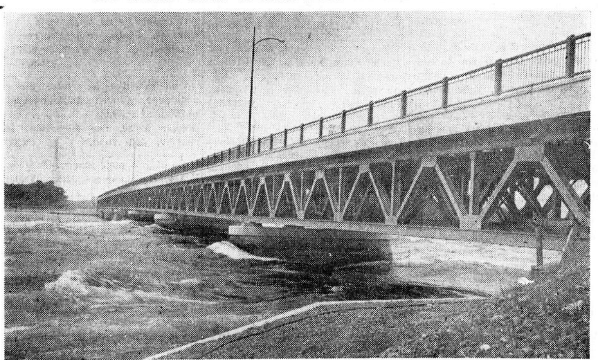
Le nouveau pont Mgr Langlois est situé dans un paysage des plus enchanteurs comme on peut le constater par cette photo saisie du côté de Côteau. Ce pont numéro deux mesure 1325 pieds de long et ses approches ne laissent certainement rien à désirer. Le coût total de la construction de ce pont ultra-moderne atteindra presque $9 millions.
