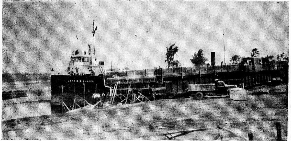
Cette photo a été saisie le jour de l'ouverture du pont samedi, le 11 septembre dernier. Les travaux sur le pont tournant, qui mesure 217 pieds, coûteront près d'un demi-million. Il devrait être complètement terminé dans un avenir très rapproché. On remarque ci-dessus un
