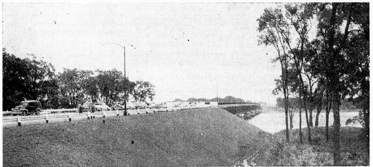
Le nouveau pont Mgr Langlois est situé dans un paysage des plus enchanteurs comme on peut le constater par cette photo saisie du côté de Côteau. Ce pont numéro deux mesure 1325 pieds de long et ses approches ne laissent certainement rien à désirer. Le coût total de la construction de ce pont ultra-moderne atteindra presque $9 millions.
