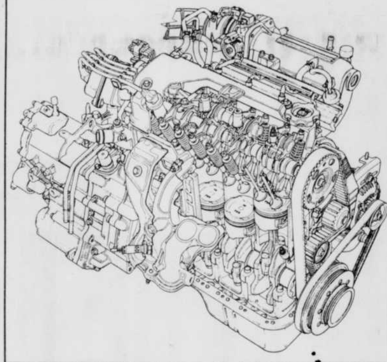
Le moteur à 16 soupapes de la Honda Civic S développe 125 chevaux.
