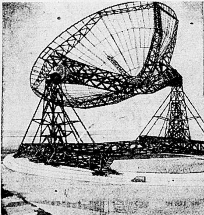
Cette autre toile d'araignée est le radio-télescope qui sera érigé à la station expérimentale de Jodrell-Bank, à Londres, tel qu'il apparaît sur un dessin à l'échelle. Le but de cette construction est de permettre aux astronomes d'obtenir des informations plus complètes sur les "radio-étoiles" mystérieuses, car, si elles nous envoient des signaux radio-électriques, elles restent invisibles à nos yeux.
