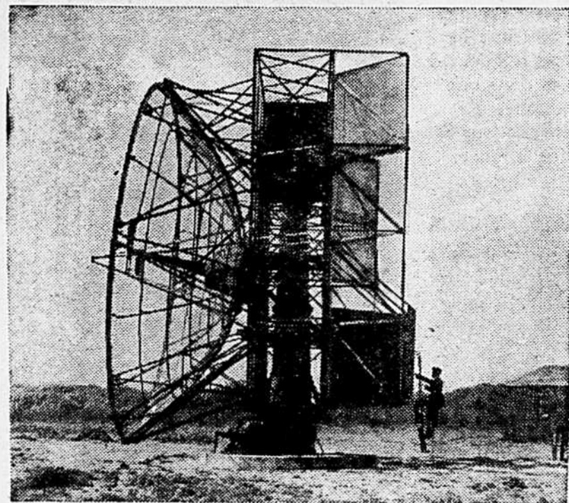
Cette antenne de radar, dont l'espèce de miroir est visiblement inspiré de la toile d'araignée, servait en Angleterre à la détection des avions ennemis, pendant la guerre. Maintenant elle sert d'aide à la météorologie, mais il a évidemment fallu étudier la construction d'appareils météorologiques pouvant fonctionner en combinaison avec le radar.
