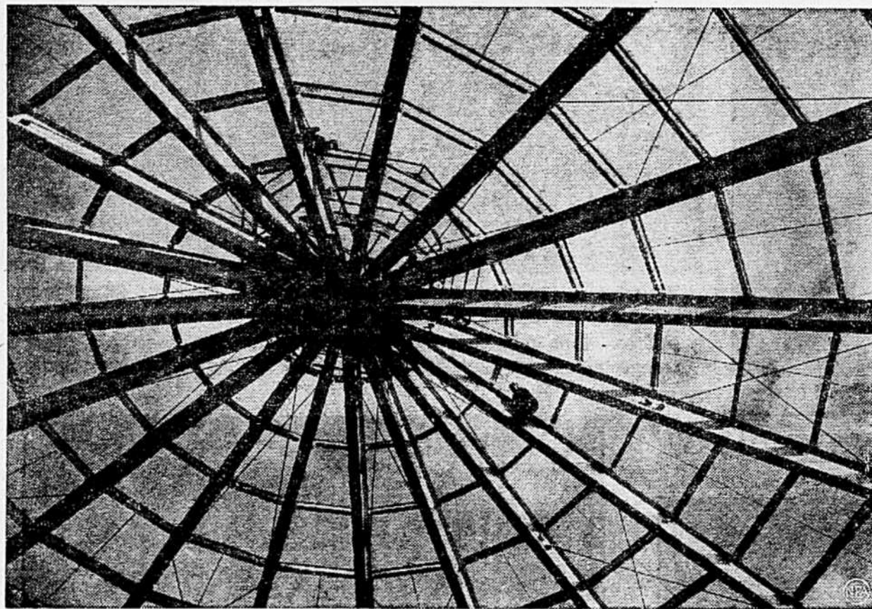
Cette immense toile d'araignée, où les hommes semblent remplir le rôle de l'araignée, n'est autre que la charpente du toit de l'édifice "B", en construction, du centre de recherche de la Ford-Motor, à Dearborn, au Michigan, où l'on étudiera divers projets concernant la défense nationale. Cette forme en "toile d'araignée" est particulièrement solide.
