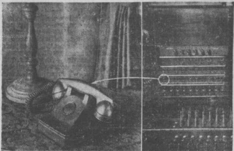
L'appareil téléphonique plaqué or dont se servira Sa Majesté, sur le convoi royal. A droite, le multiple qui servira de liaison téléphonique aux différentes parties du convoi. Le cercle indique la sortie du téléphone qui servira à l'appareil plaqué or.
