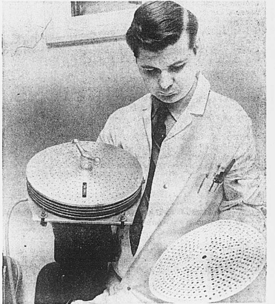
Cet appareil est utilisé pour déterminer la grosseur des poussières en suspension, après quoi on en détermine la composition. Les petites particules sont jugées plus nocives en raison de la possibilité qu'elles ont de s'infiltrer dans les poumons.
