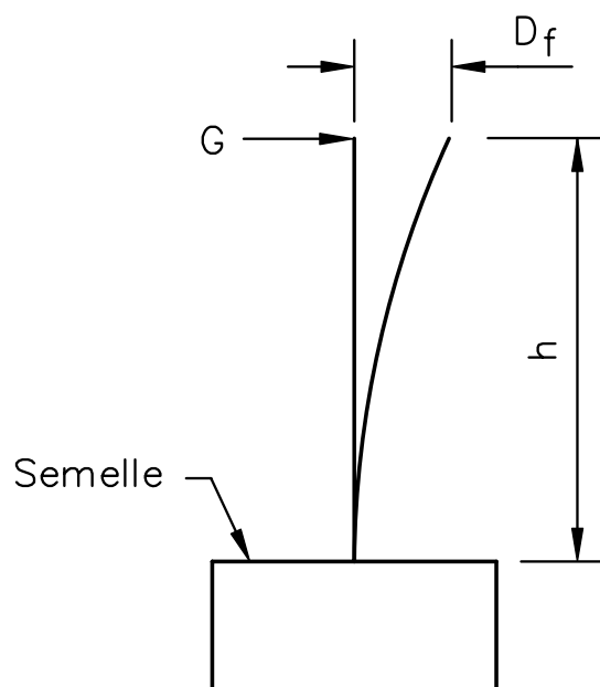
Figure 11.1-1 Déplacement du point d'appui fixe
