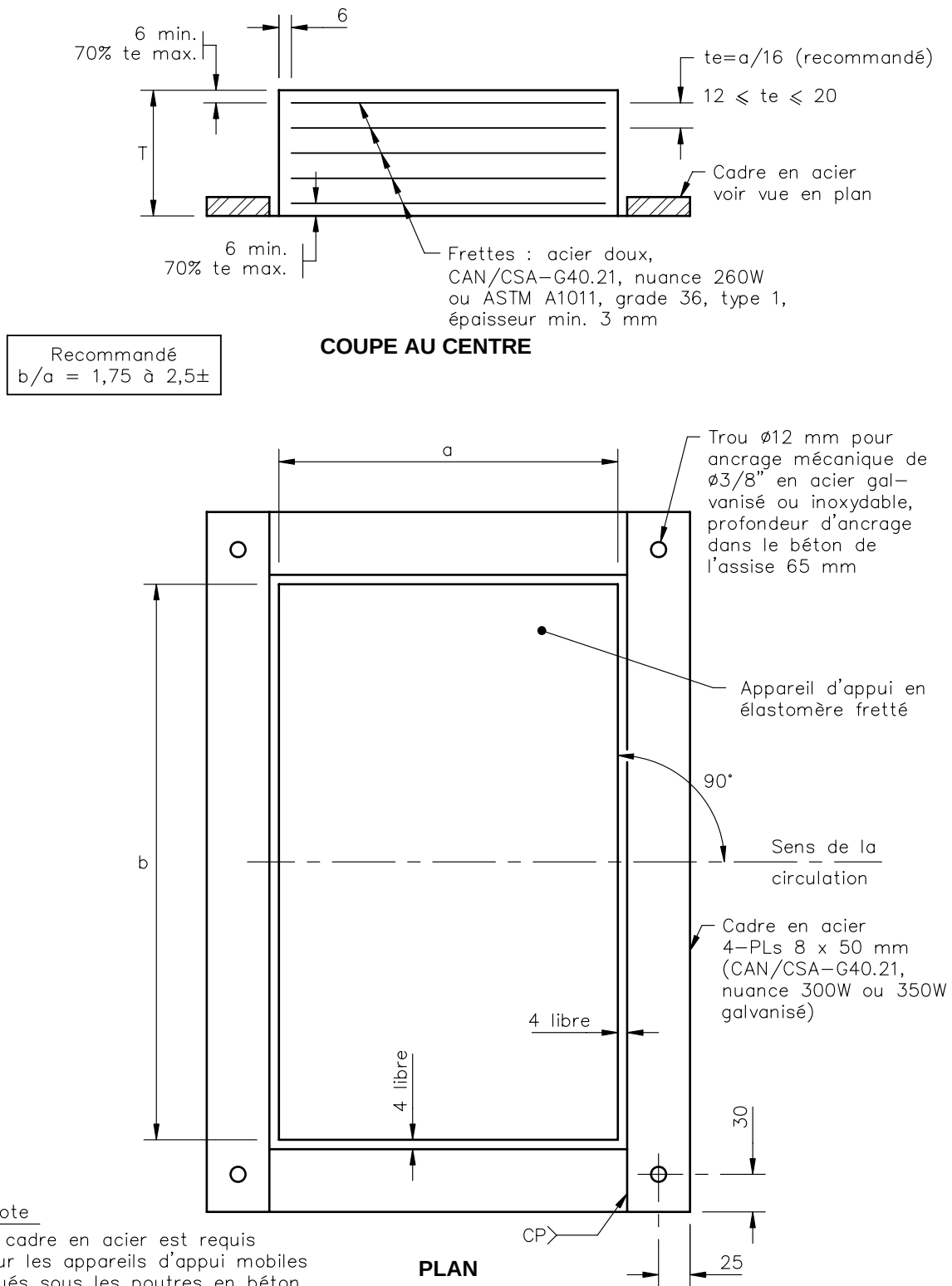
Figure 11.2-1 Appareil d'appui en élastomère fretté
