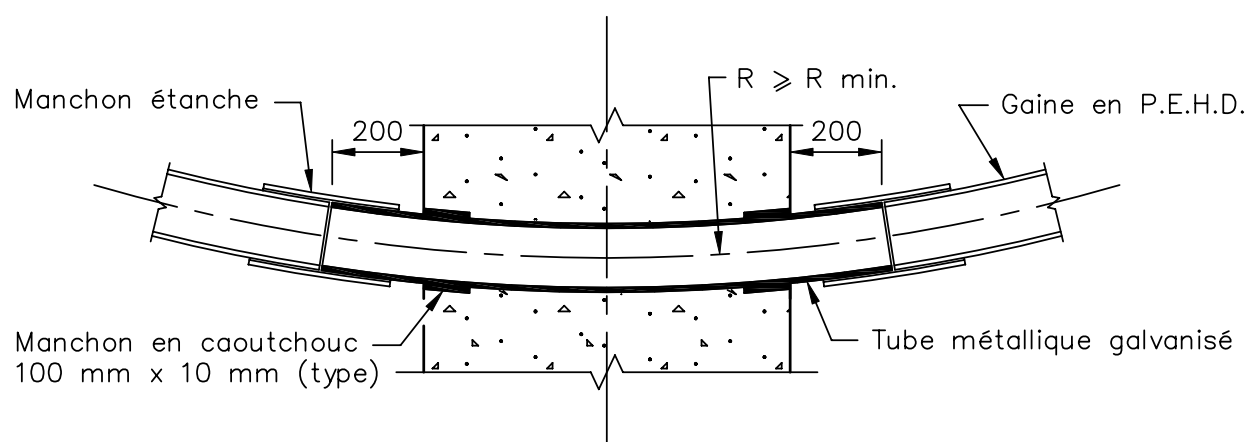
Figure 8.3-1 Déviateur simple
