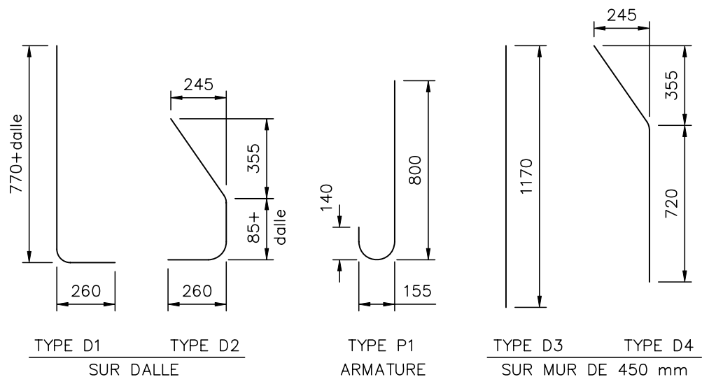
Figure 12.2-6 Glissière en béton type 201
