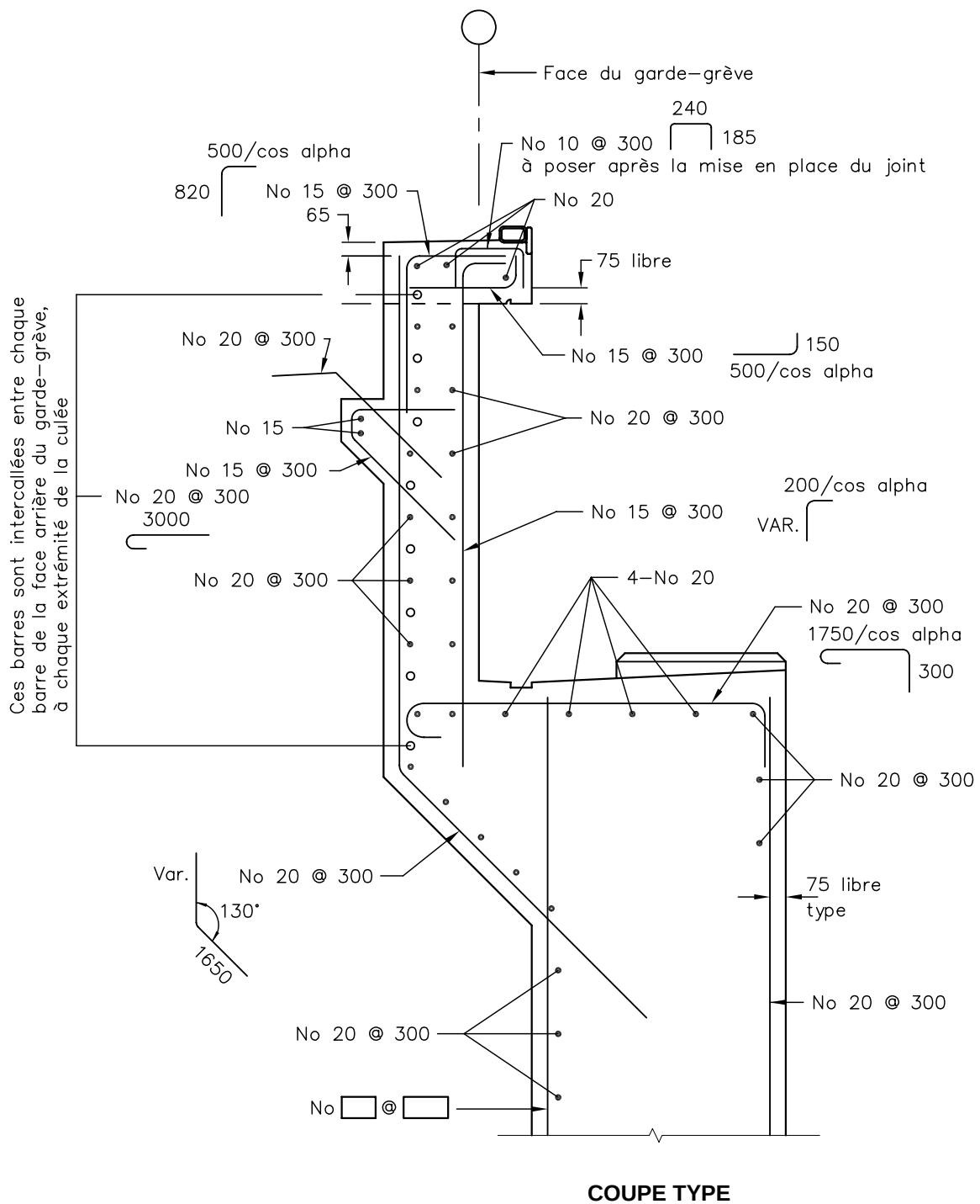
Figure 11.3-6b Culée-galerie avec joint de tablier HSS (armature)
