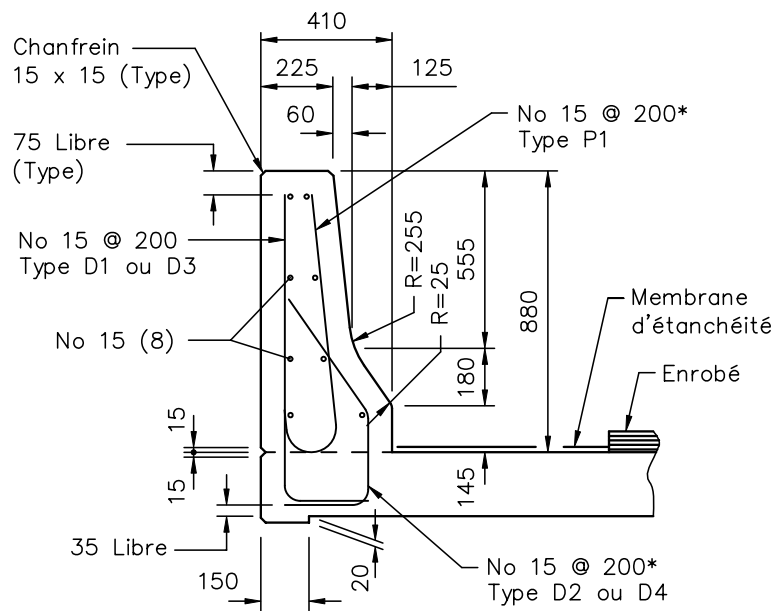
COUPE TYPE (Dalle sur poutres)
