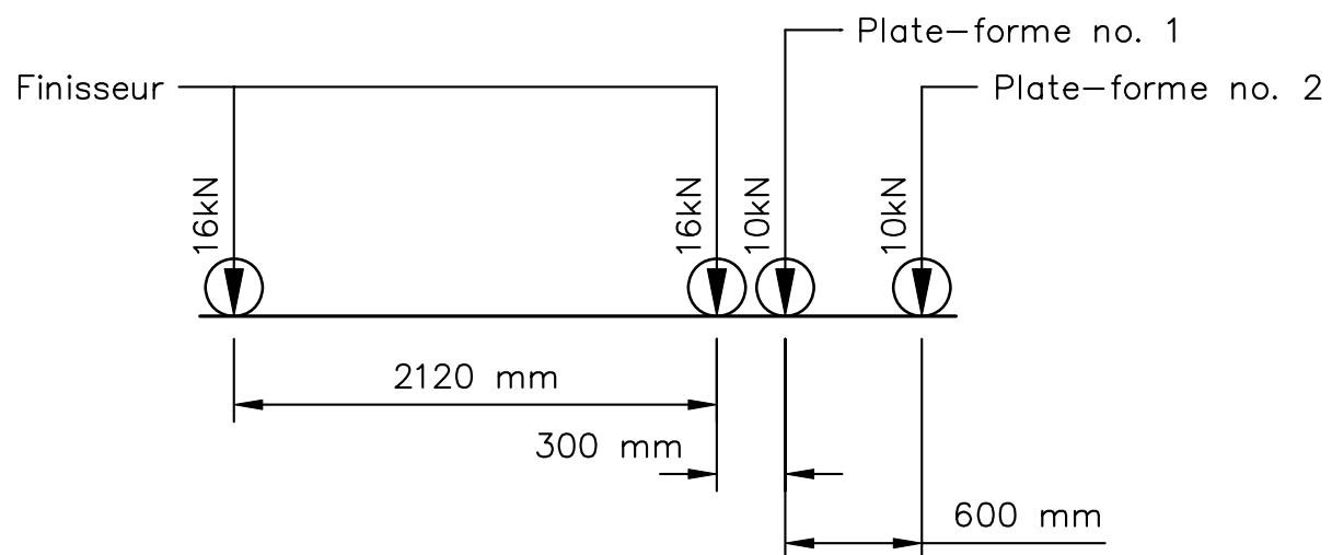
Figure 3.3-3 Train de charges mobiles minimales par extrémité (Finisseur automatique et plates-formes de travail)
