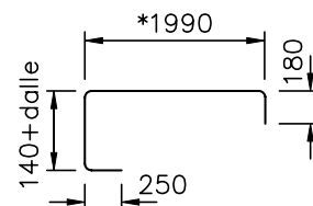
ARMATURE TYPE T2 SUR DALLE ÉPAISSE
