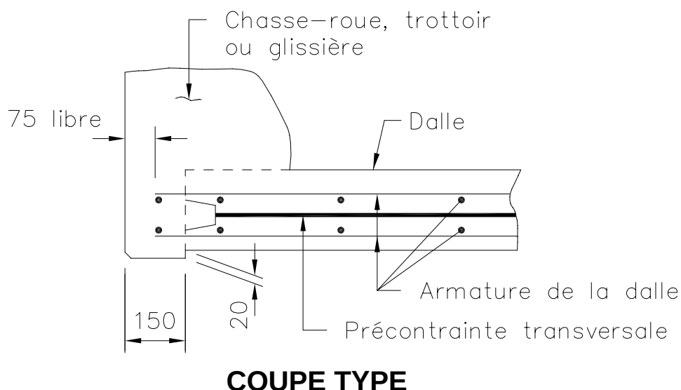
Figure 8.3.3 Précontrainte transversale
