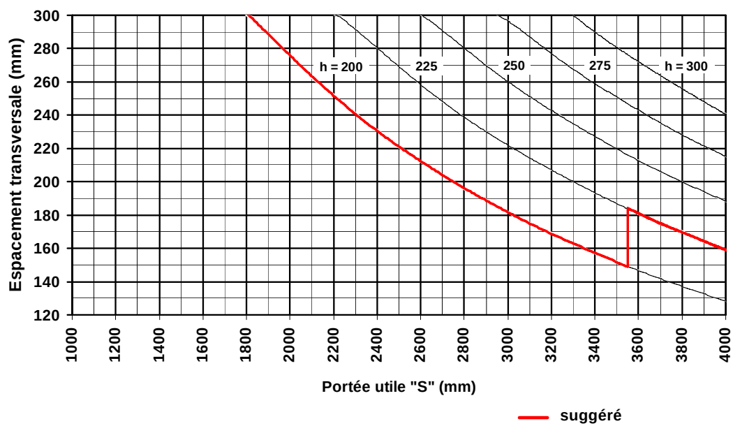
Figure 8.2-3 Armature principale N° 20
