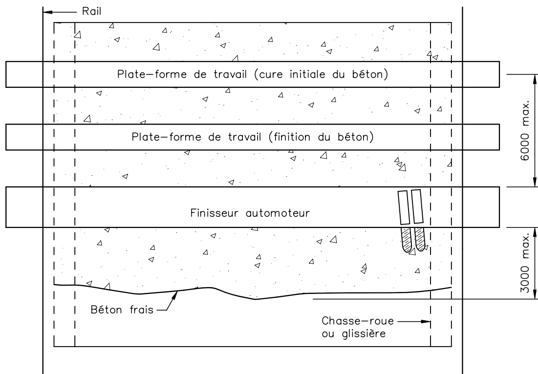
Figure 3.3-2 Disposition du finisseur automatique et des plates-formes de travail
