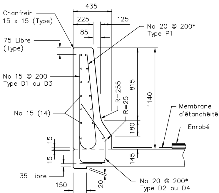
COUPE TYPE (Dalle sur poutres)
