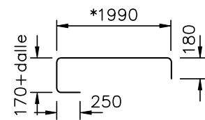
ARMATURE TYPE T1 SUR DALLE SUR POUTRES
