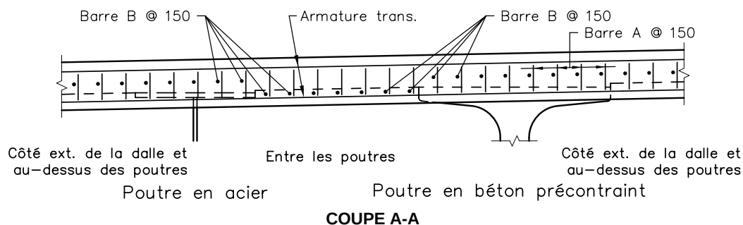
Figure 11.3-9b Détail de l'extrémité de la dalle avec joint de tablier HSS
