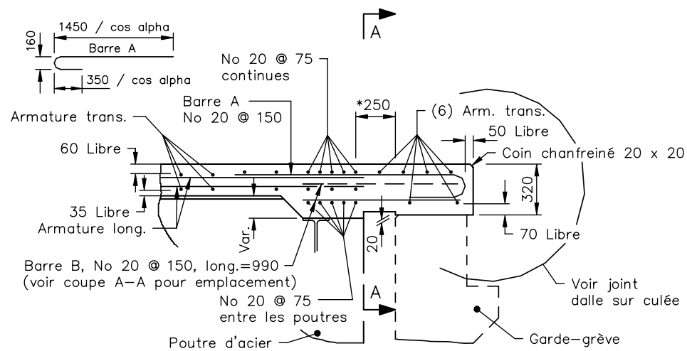
PROFIL - POUTRE EN ACIER
