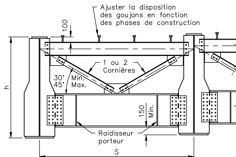
Figure 10.6-2 Contreventement en K aux appuis
