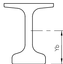
Figure 8.3-5 Caractéristiques des poutres préfabriquées de type NEBT
