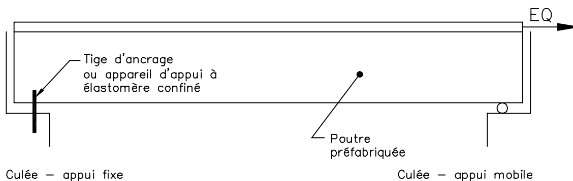
Figure 8.3-16 Stabilité longitudinale
