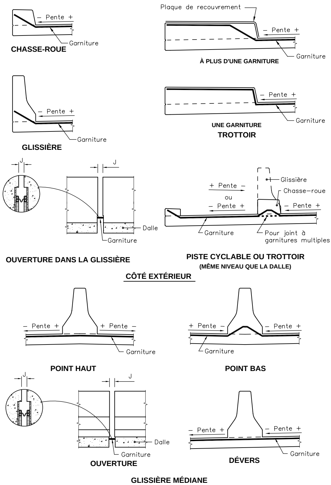
Figure 11.3-14 Profil de la garniture en élastomère
