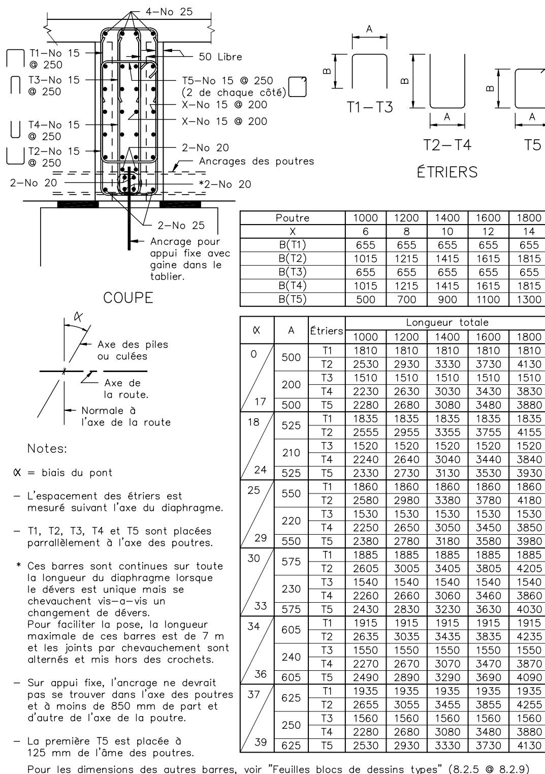
Figure 8.2-8 Diaphragme sur pile – Tablier continu
