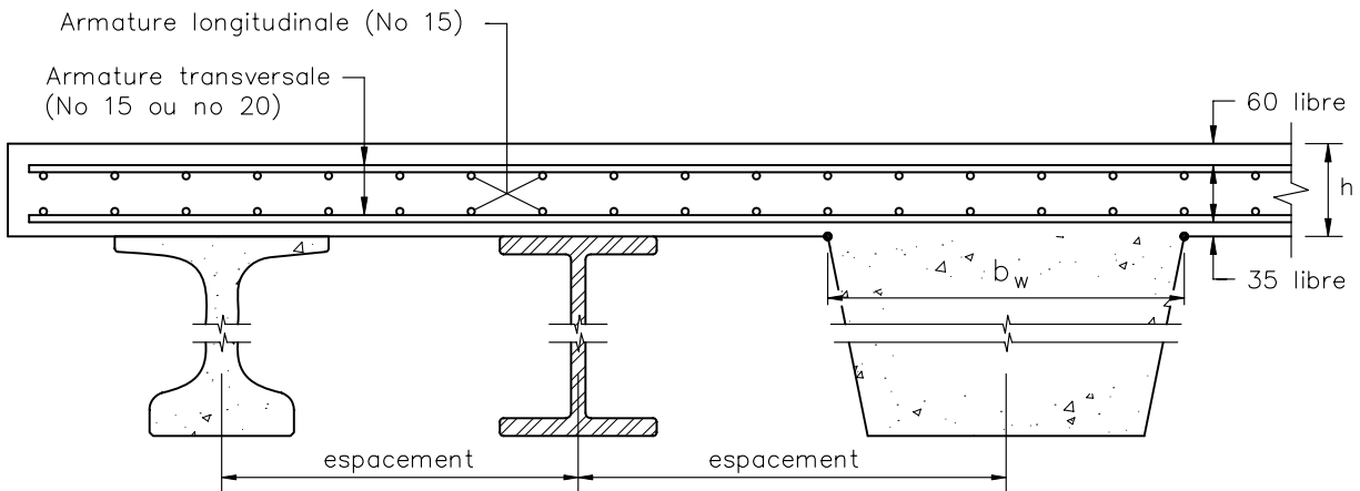
Figure 8.2-1 Disposition de l'armature
