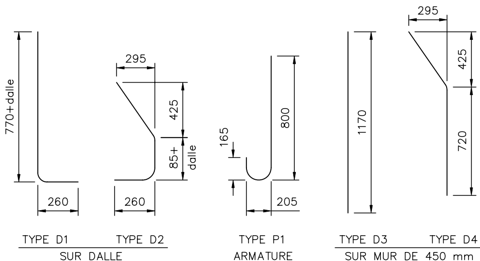
Figure 12.2-12 Glissière en béton type 311B
