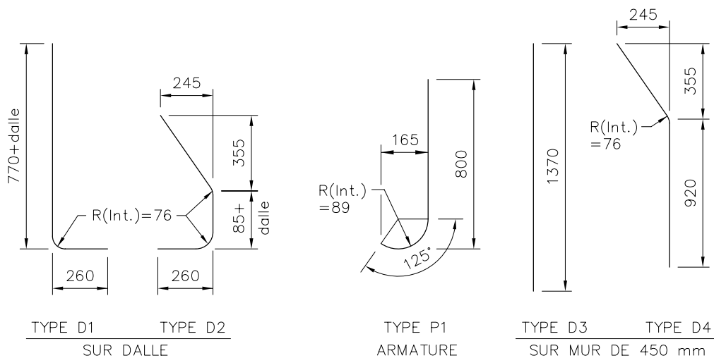
Figure 16.4-1 Glissière 201 en béton renforcée à l'aide d'armatures en matériaux composites
