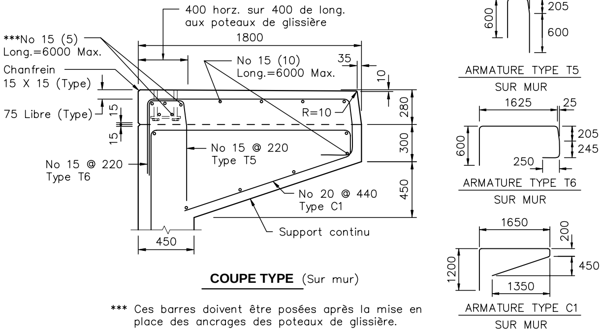
Figure 12.2-3 Trottoir non séparé de la chaussée
