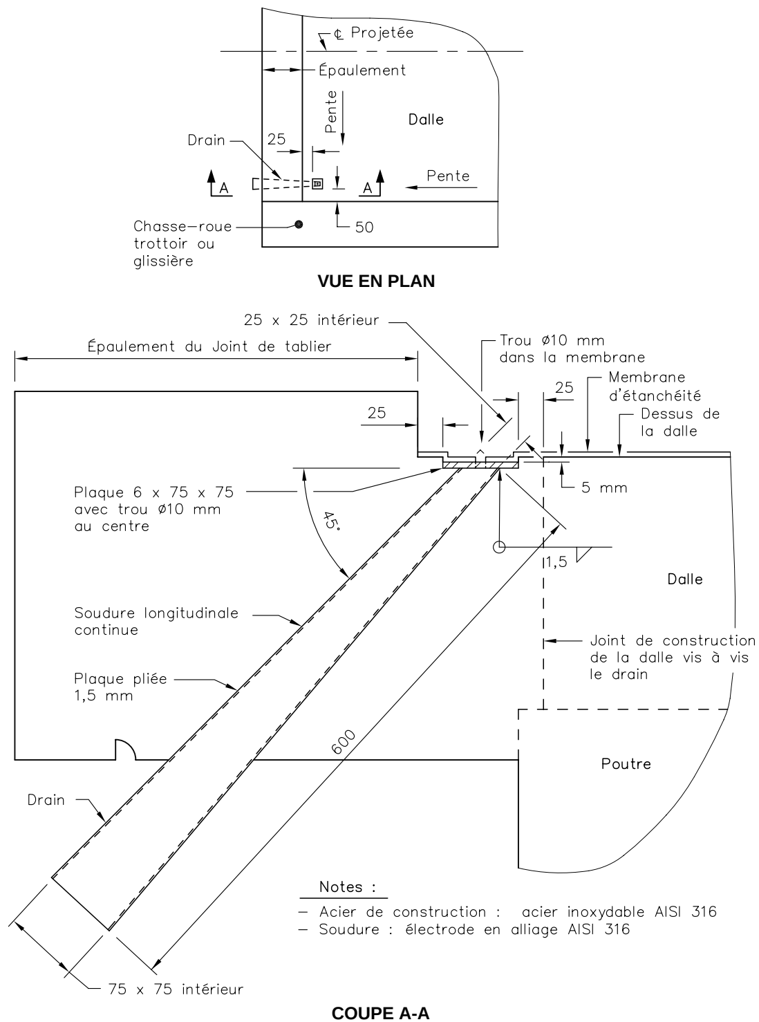
Figure 2.2-2 Drain d'interface
