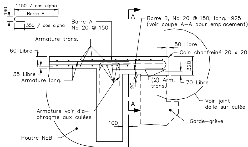
PROFIL - POUTRE PRÉFABRIQUÉE EN BÉTON PRÉCONTRAINT
