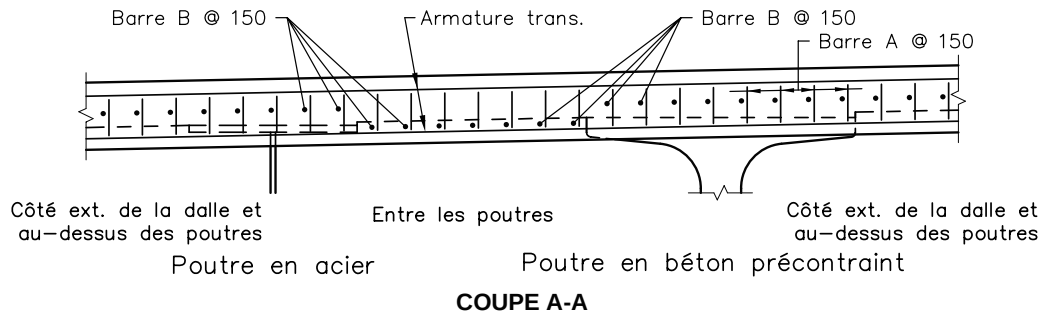
Figure 11.3-9a Détail de l'extrémité de la dalle avec joint de tablier conventionnel
