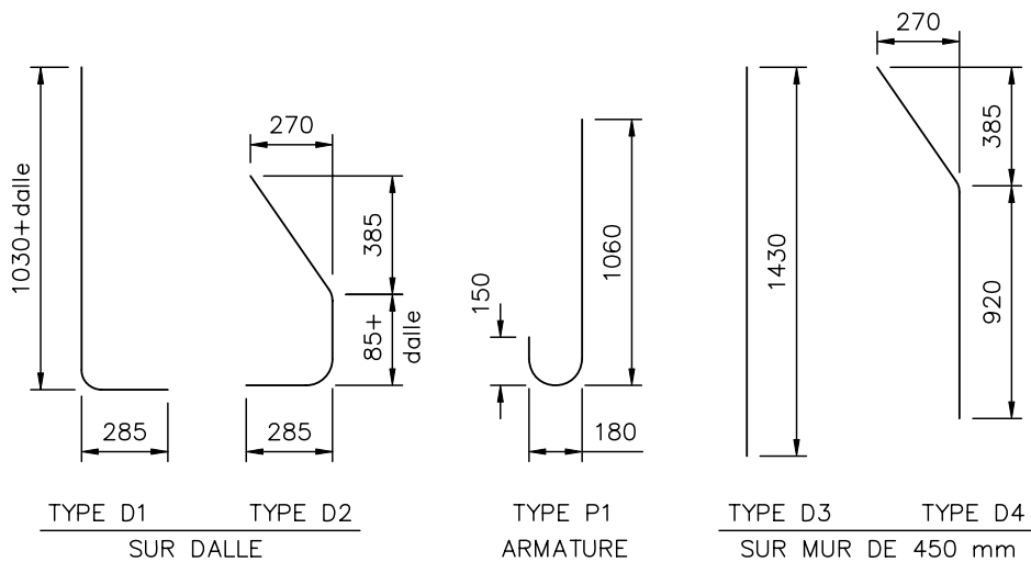
Figure 12.2-11 Glissière en béton type 301
