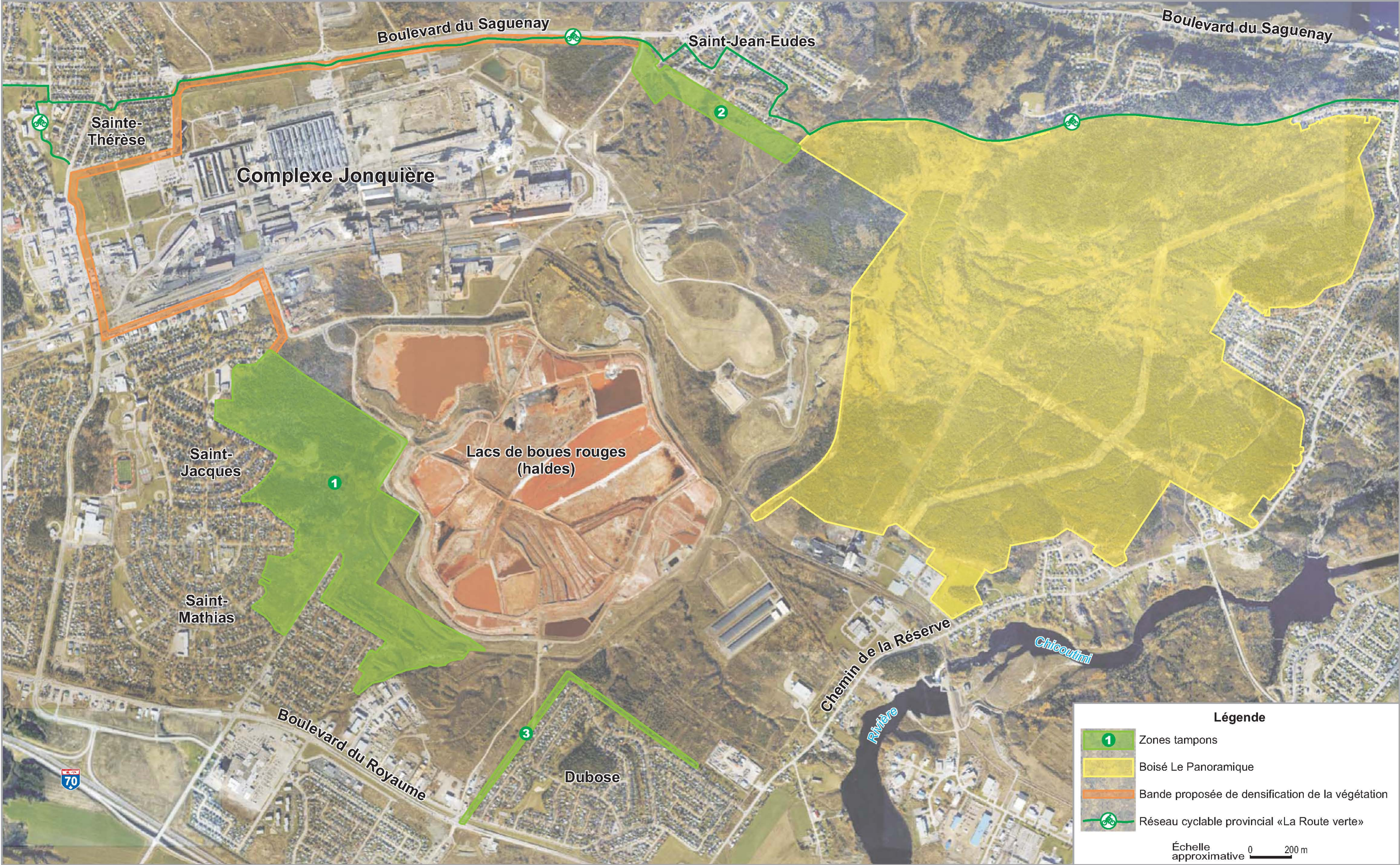
Figure 6 La ceinture verte du projet AP50 (AP60) du complexe Jonquière
