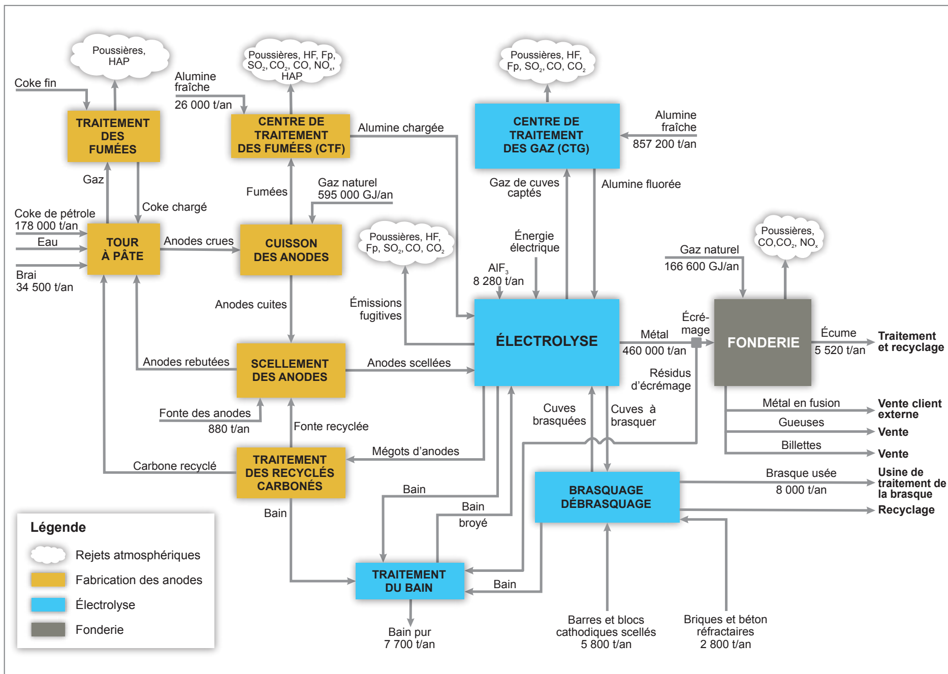
Figure 3 Le schéma de procédé et les flux de matières de l'usine AP50 (AP60) du complexe Jonquière
