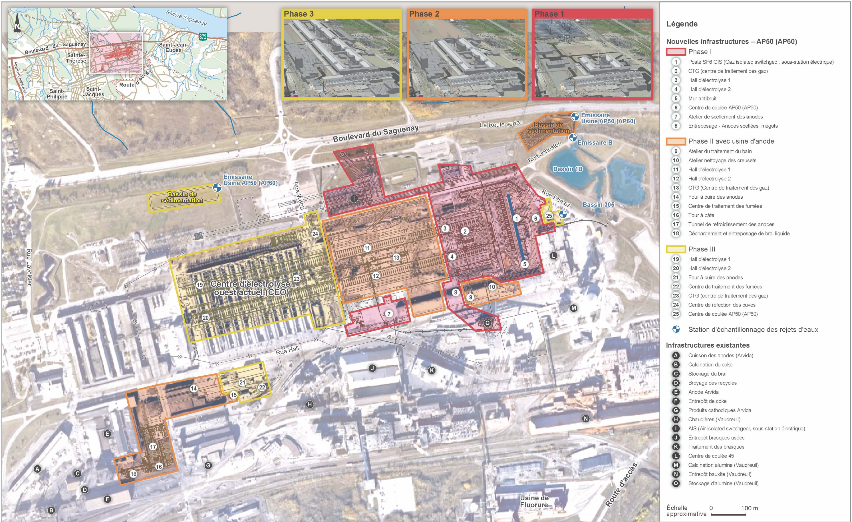
Figure 2 Les phases de construction de l'usine AP50 (AP60) du complexe Jonquière
