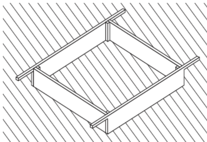
Figure 2 – Contenant sans fond de dimension intérieure de 1\text{ m} \times 1\text{ m} \times 0,25\text{ m}
