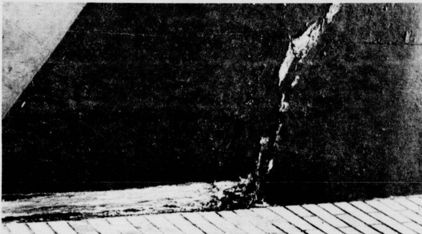
Une autre fissure qui n'a rien d'élégant. Toutefois, placée dans un coin, elle ne dépare pas trop le paysage. Est-ce vraiment la dynamite qui a provoqué cette fissure ou bien la qualité du béton ou encore son épaisseur?
