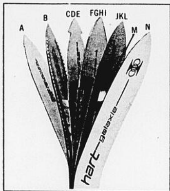
Cette coupe révèle la construction interne de la plupart des skis Hart
