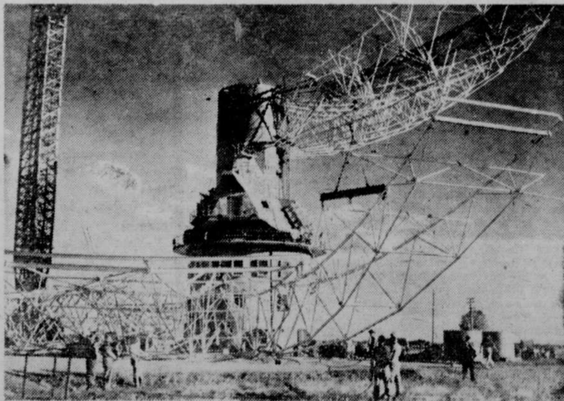
La tourelle tournante étant installée sur sa tour de béton armé, les éléments en acier sont mis en place.
