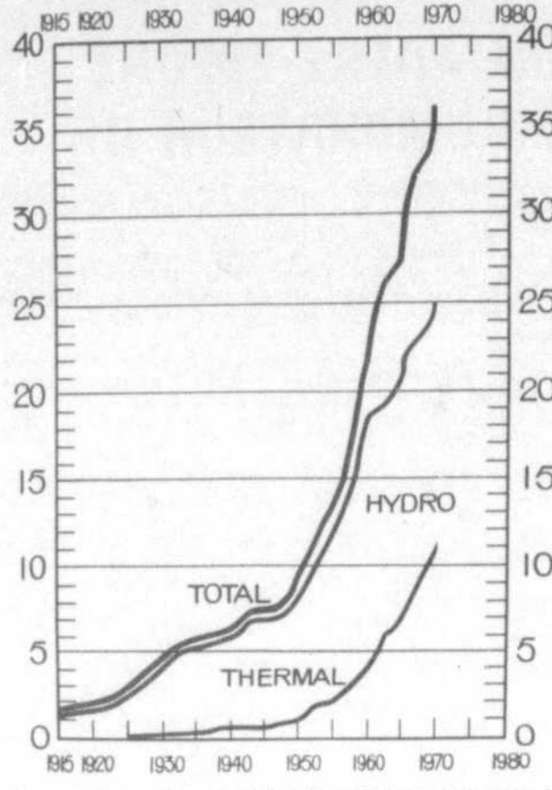
La vignette ci-dessus reproduit la croissance de la capacité génératrice d'énergie électrique au Canada, de 1915 à 1980. On peut constater que les progrès furent particulièrement marqués depuis 1950. Cette vignette nous a été fournie par l'Association Canadienne de l'électricité.
