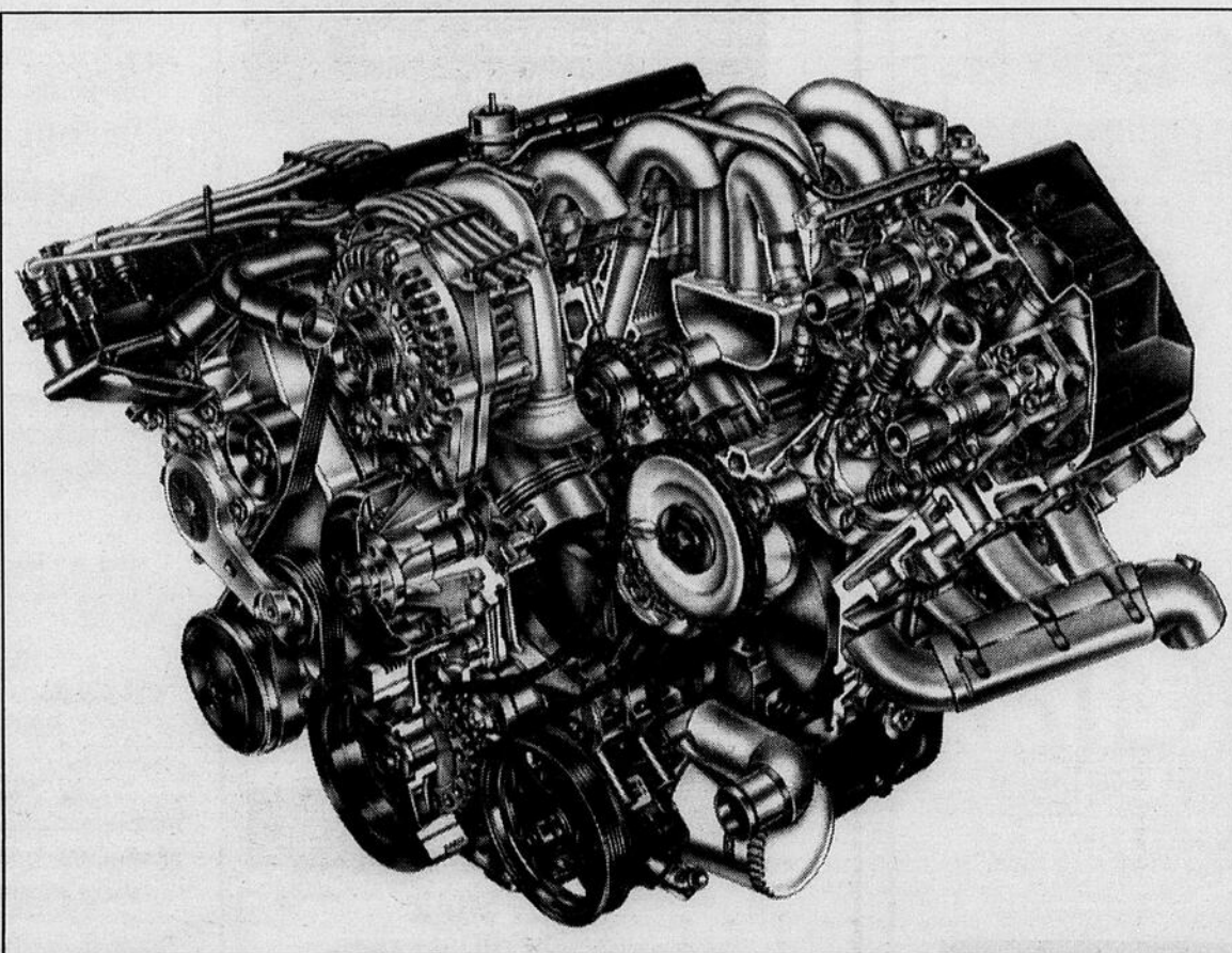
Le nouveau moteur V8 de 4,6 litres de la Lincoln Mark VIII possède deux arbres à cames en tête et son bloc comme sa culasse est en aluminium. Il s'agit du premier V8 multisoupapes à jamais être construit en série par Ford. Il développe 280 chevaux, soit 33 % de plus que la livrée à deux soupapes par cylindre qui en délivre 210.
