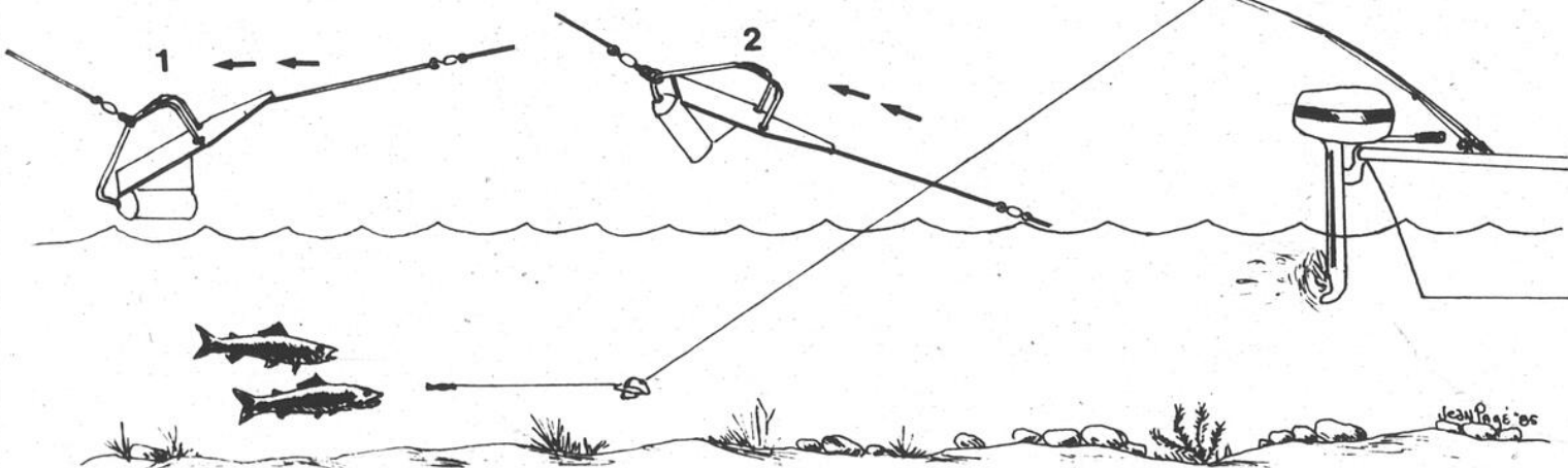
1) Dans sa position de plongée, le "planeur" maintient le leurre à la profondeur désirée. 2) Etant désengagé, il se remonte facilement, en surface, offrant peu de résistance au pêcheur, qu'il y ait ou non un
