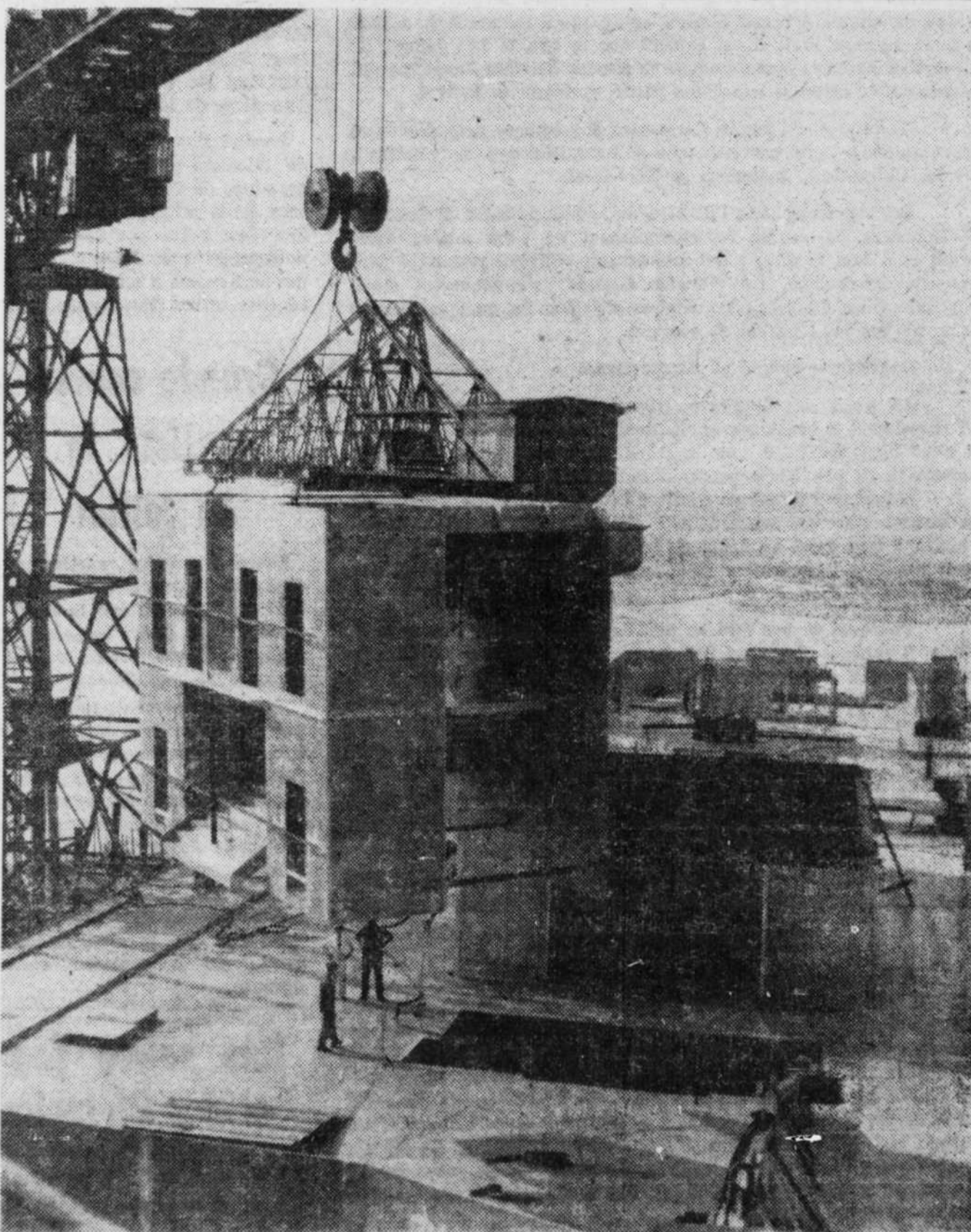
LA STRUCTURE DE L'ORIANA, pour ce qui est reté si grande de ce métal. C'est un autre avantage des sections en aluminium, a pu être préfabriquée, dont on tire profit dans les chantiers navals, assemblée et soudée aux ateliers, grâce à la légè-
