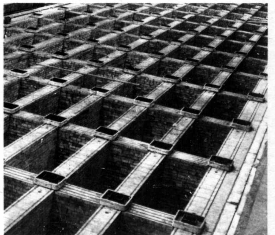
IL AURA FALLU 200 wagons de briques et quatre mois à une centaine d'hommes pour construire les différentes sections de la nouvelle fournaise à électrodes à l'Alcan d'Arvida.
