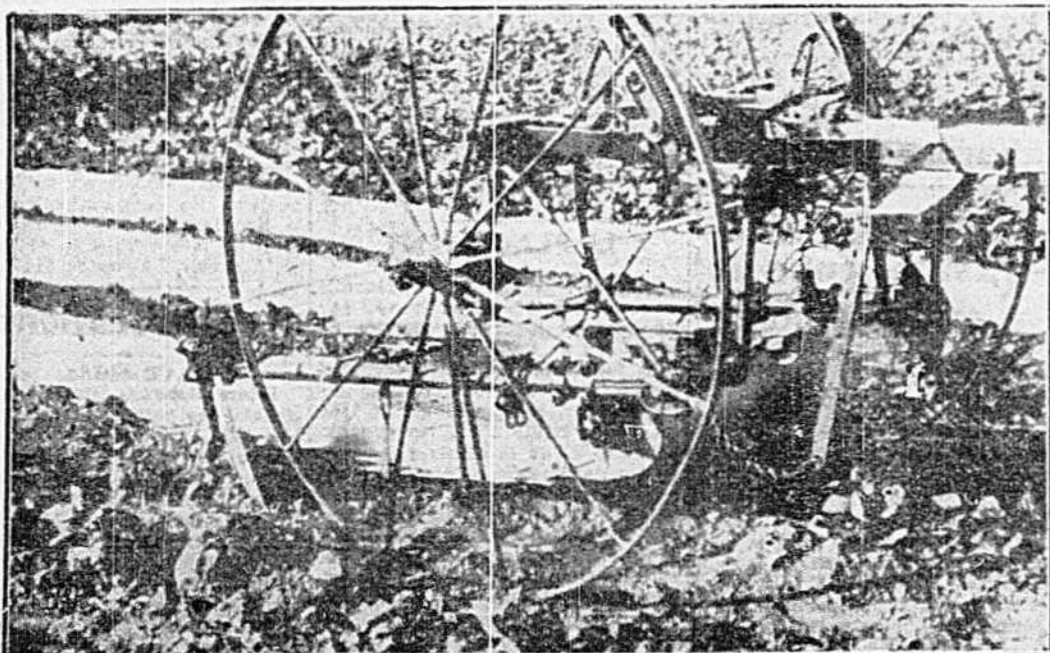
Cet appareil est l'invention de M. Alfred Pfeiffer, de San Antonio, vendeur de chaussures. L'on est d'avis que cette invention sauvera des milliers de dollars aux fermiers annuellement. Cette machine répand des lisières de papier sur les produits de la ferme quand il y a danger des gelées. Jusqu'à présent, le cultivateur était contraint de recouvrir ses légumes de terre, ce qui lui occasionnait une dépense variant entre vingt et trente dollars de l'acre. Pfeiffer prétend qu'à l'avenir les fermiers pourront s'en tirer avec une dépense d'environ dix dollars l'acre.
