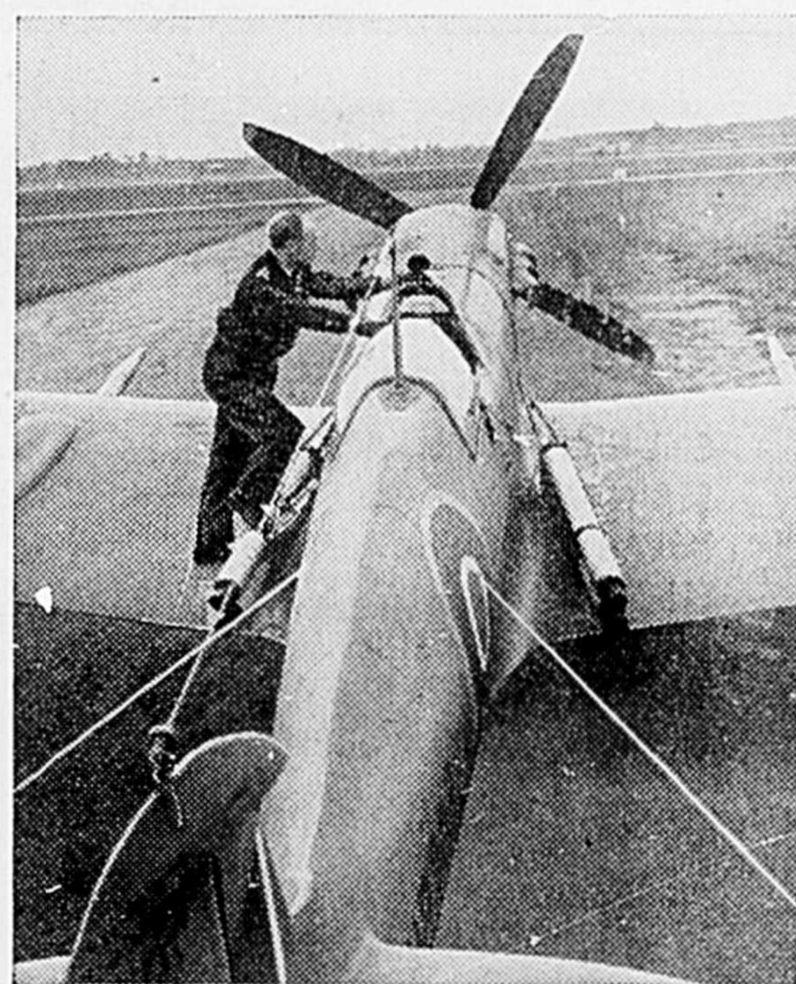
Les fusées servent au lancement des avions à bord des porte-avions britanniques. Elles sont montées de part et d'autre du fuselage. Elles augmentent l'accélération au départ et réduisent la distance nécessaire au décollage. Leur action dure quatre secondes, après quoi elles tombent à l'eau. Sur la photo, un pilote monte dans son "Spitfire" que des fusées aideront à décoller.
