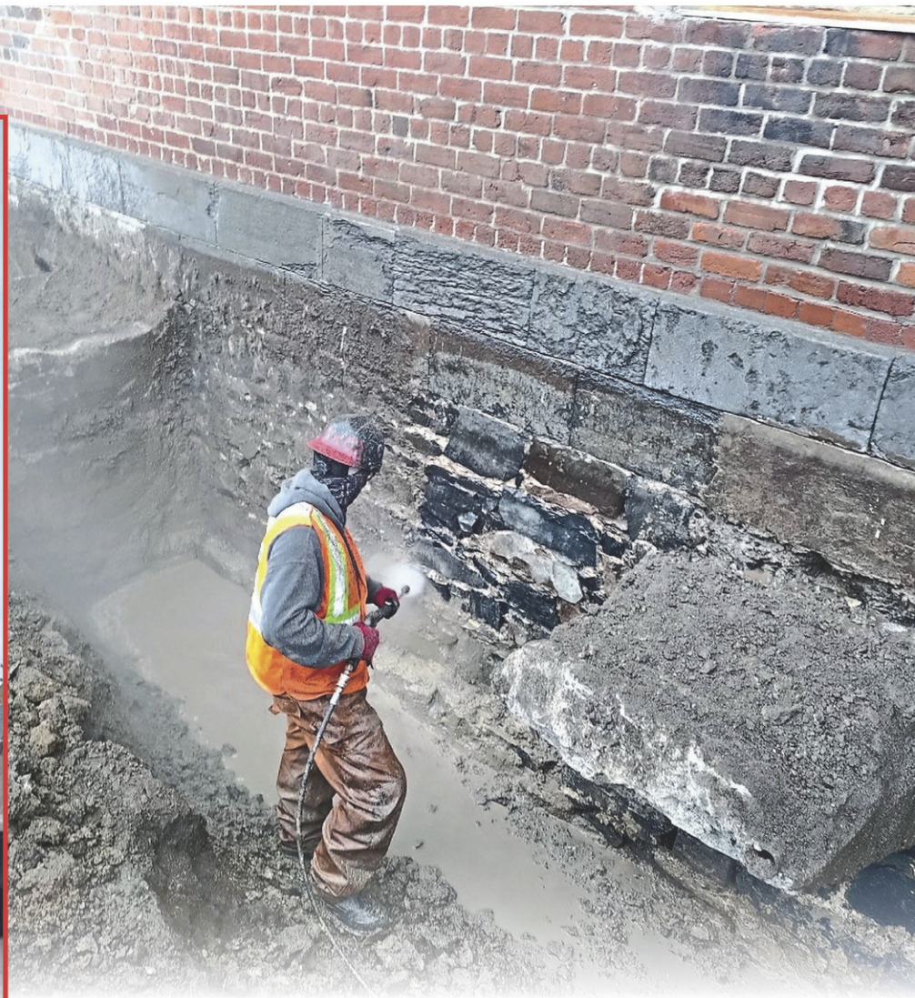
La fondation a été nettoyée pierre par pierre pour ne pas compromettre l'adhérence. Il va de soi que, durant ce processus, la température doit être des nôtres.
