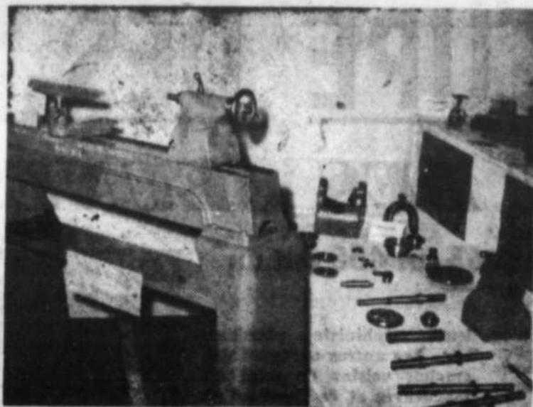
Tour à bois dont le modèle, les pièces coulées et le montage sont entièrement l'oeuvre d'élèves de l'Ecole Technique de Montréal.
