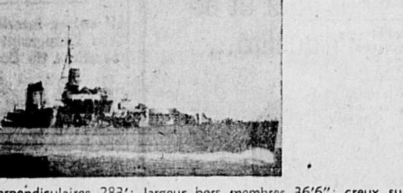
DESCRIPTION: Longueur hors tout 301'6"; largeur entre les perpendiculaires 283'; largeur hors membrures 36'6"; creux sur quille (jusqu'au pont supérieur) 17'6". Tonnage brut 1510. MACHINES: à vapeur, triple expansion, hélices jumelles, 5500 c.v. indiqués. Deux (2) chaudières tubulaires et trois tambours. Peuvent être transformés en cargos, passagers ou navires frigorifiques. LIEU: Shelburne, N.-E. et Vancouver, C.-B. PRIX de $80,000.00 à $140,000.00 (Chacun) selon leur état.
