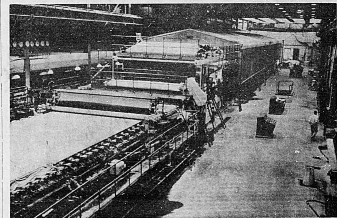
Voici la fameuse machine à papier Millspauh dans toute sa grandeur. Elle mesure 325 pieds de longueur et peut produire 100 tonnes de papier par jour. Cette machine vaut environ 2 1/2 millions.
