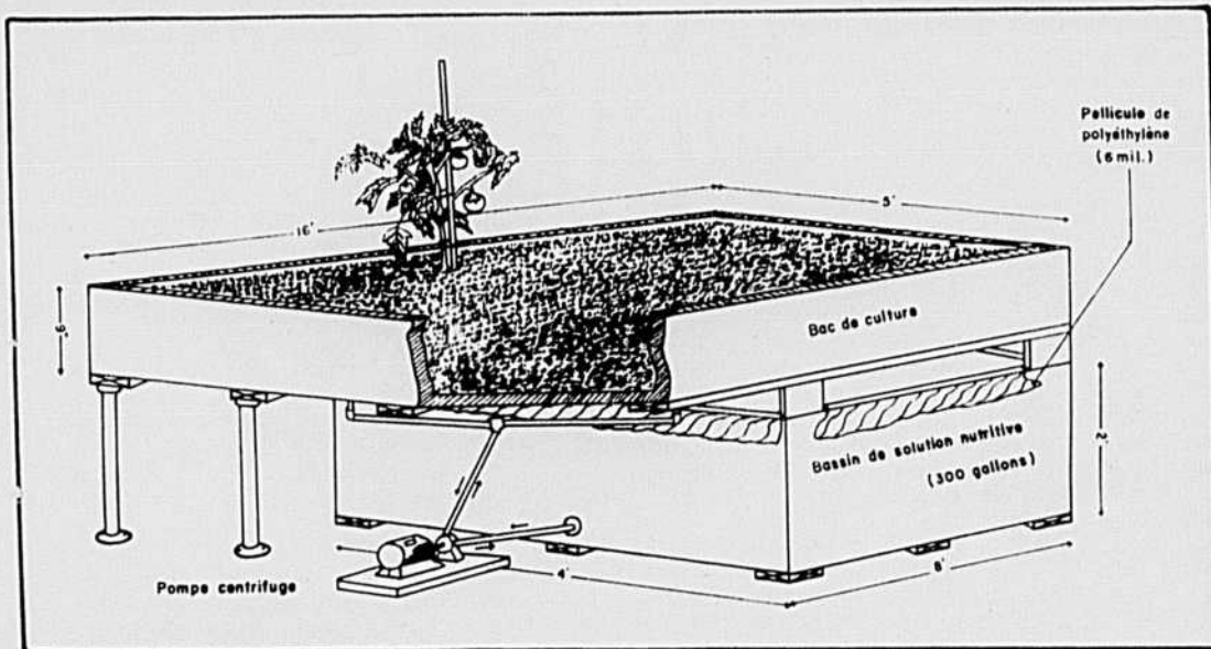
Croquis schématique illustrant une installation pour la culture sans sol.
