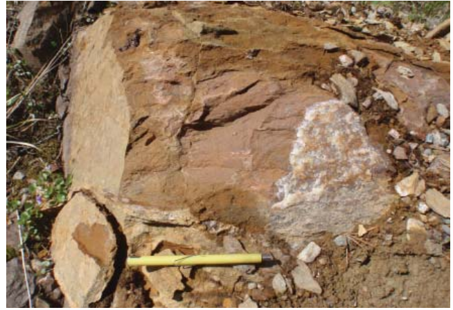
PHOTO 2 - Coulée massive de basalte fortement ankéritisée. Formation de Clermont-Disson (Ac1). Affleurement 12-PL-1050 (655964E, 5432244N).
