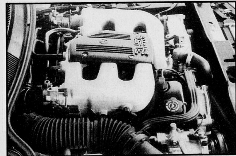
Le moteur de la Vision est un V6 de 3,5 litres 24 soupapes délivrant une puissance de 214 chevaux.
