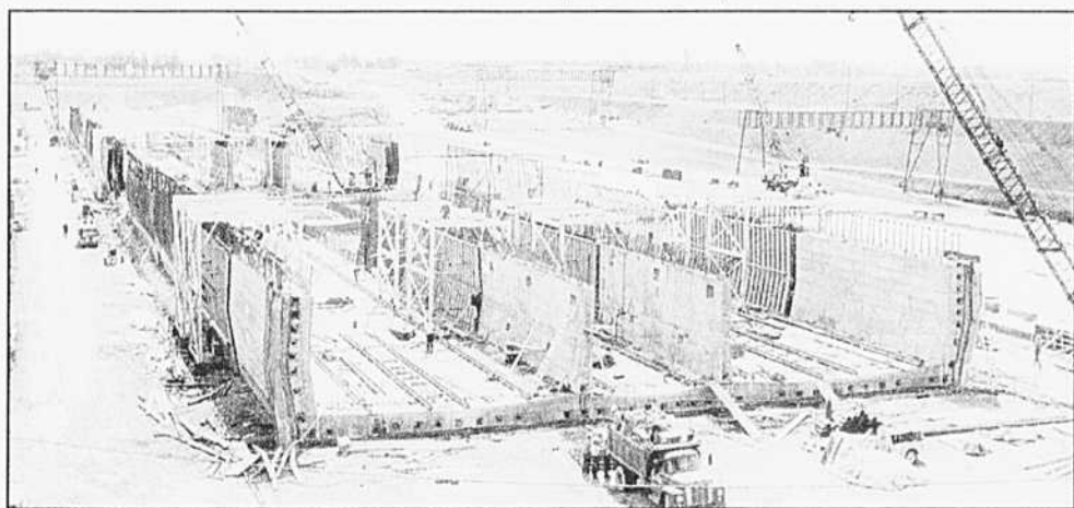
Construction du pont-tunnel Louis-Hippolyte-La Fontaine - Cale sèche, vue de l'extrémité nord-est, 30 juillet 1964. Il fallait deux semaines pour couler entièrement la structure de 32 000 tonnes au fond du fleuve... (Photo d'archives - Ministère des Transports du Québec)
