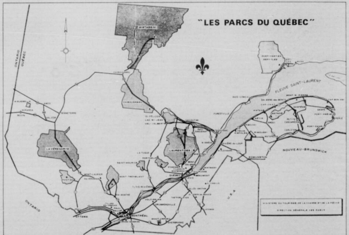
Cette carte publiée par le ministère du Tourisme, de la Chasse et de la Pêche du Québec indique où sont situés les magnifiques parcs de la Belle province.
