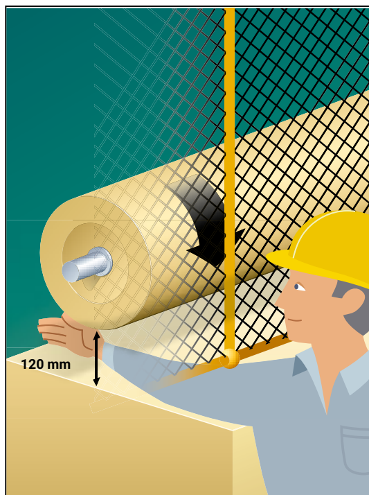
Figure 37. Prévention à l'étape de la conception pour un cylindre et une partie fixe
