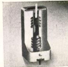
TRANSFORMATEUR F.I. À NOYAU DE MAGNÉTITE
