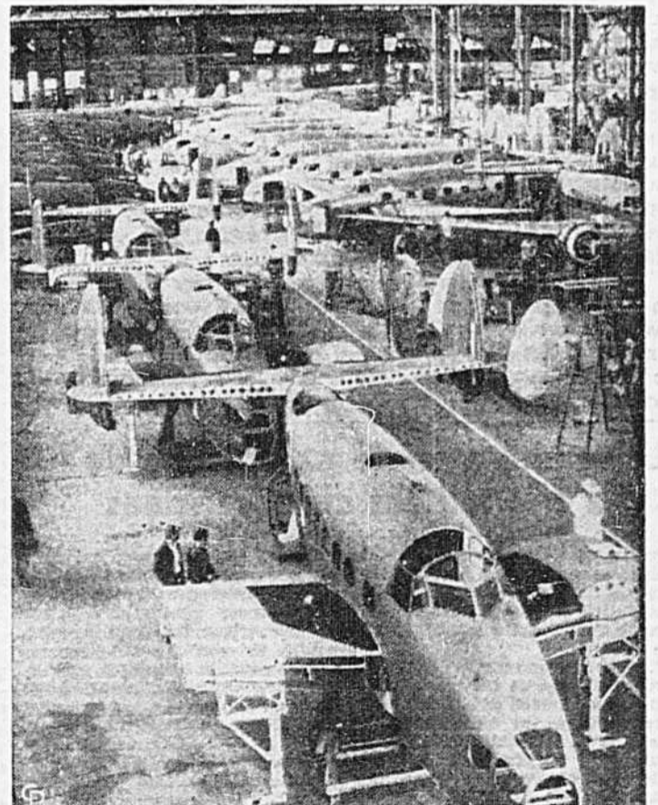
Les usines de Lockheed Aircraft Co. à Burbank, Californie, où l'on fabrique les fameux bombardiers Hudson. C'est à bord d'un de ces appareils que trois personnes ont été tuées hier à St-Hubert.
