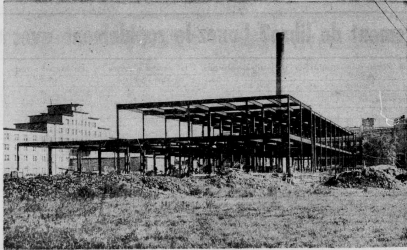
Structure métallique de la future buanderie de l'Hôpital de l'Enfant-Jésus.
