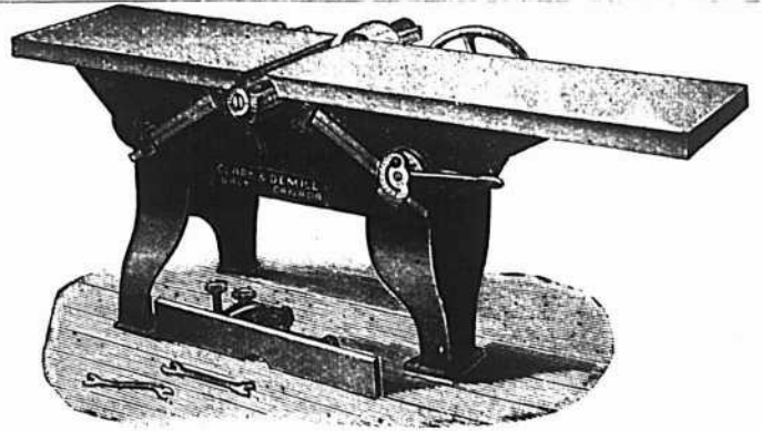
Machine "Perfection Buzz" à Blanchir et à Embouvetter Prix et descriptions envoyés avec plaisir — sur demande CLARK & DEMILL. Fabricants de grosse machinerie — garantie — pour Moulins à Scie, GALT CANADA.
