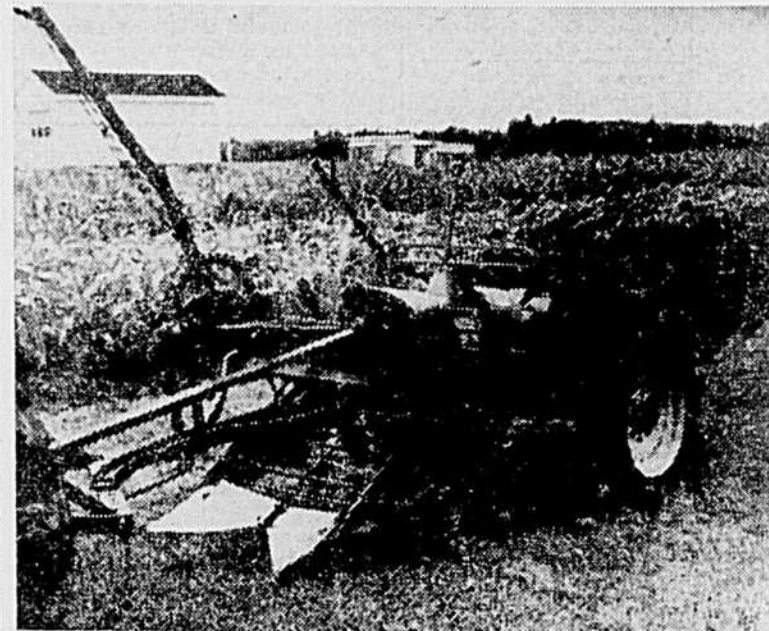
Une arracheuse de patates chez M. Paul Robitaille, de Mont-Carmel. Le sol à double tranchant a été conçu et imaginé par M. Robitaille qui l'a fait forger spécialement pour lui. Ce soc couperait moins de patates que les autres.
