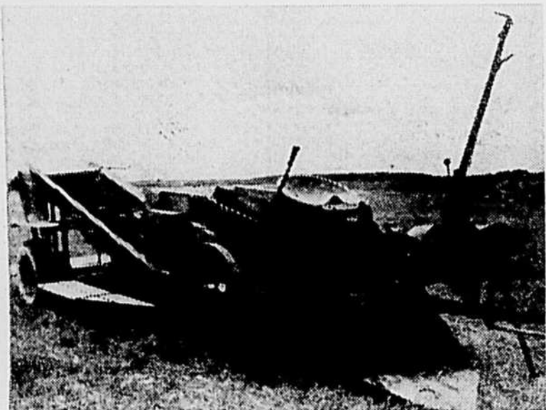
Une arracheuse-ensacheuse combinée de pommes de terre chez M. Ernest Cardinal, à Ste-Brigitte des Saulls.
