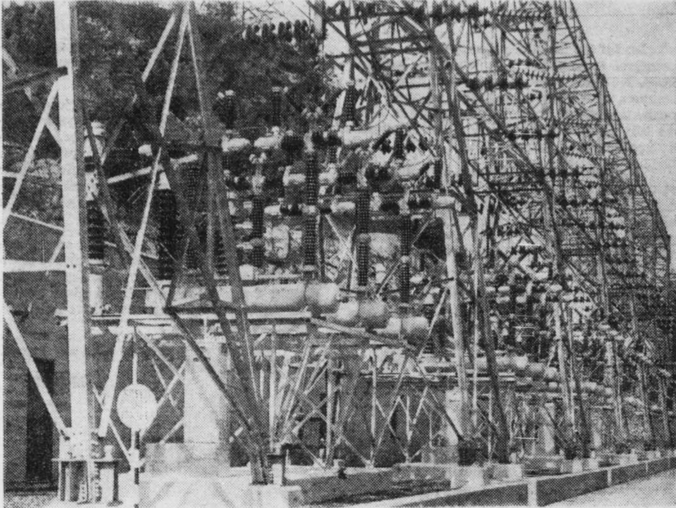
CETTE MAGNIFIQUE INSTALLATION a été faite en février et mars 1961, à l'usine hydroélectrique de l'ALCAN, à Shipshaw. Ce sont les six nouvelles unités d'interrupteurs de circuit d'énergie électrique, lesquels sont maintenant actionnés à l'air.
