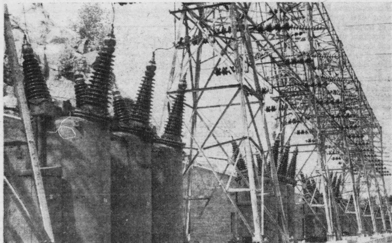
CETTE MAGNIFIQUE INSTALLATION a été faite en février et mars 1961, à l'usine hydroélectrique de l'ALCAN, à Shipshaw. Ce sont les six nouvelles unités d'interrupteurs de circuit d'énergie électrique, lesquels sont maintenant actionnés à l'air.
