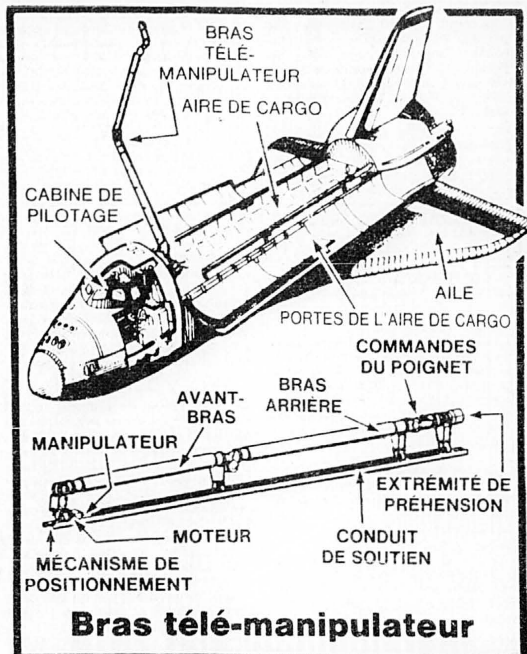
Photo UPI Le bras télé-manipulateur mis au point par le Canada sera du deuxième voyage de Columbia dans l'espace et subira des tests de fonctionnement dans le vide. Ce dessin montre où le bras est rattaché à la cabine de la navette et ses principales parties constituantes.
