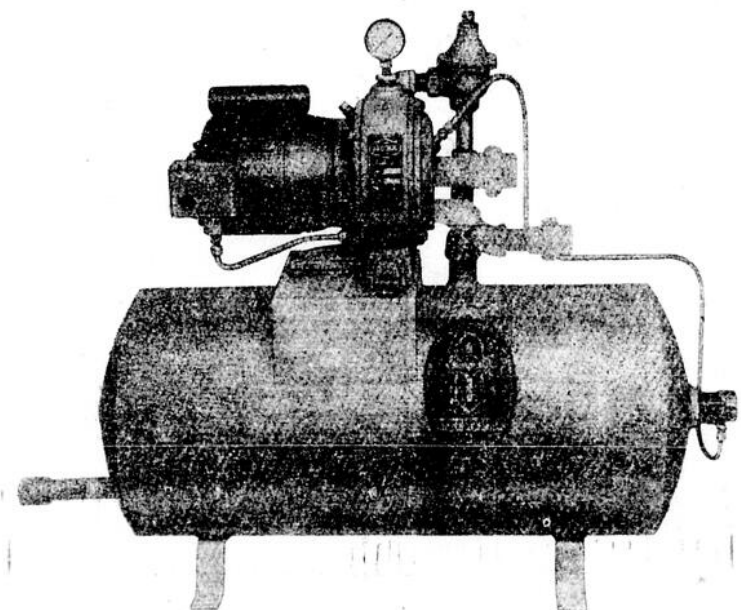
Modèle de pompe à turbine fabriquée par la National Electric
