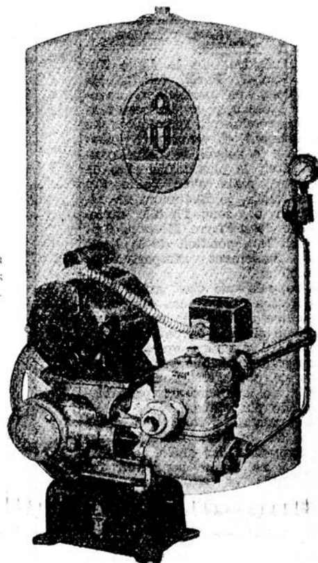
Système de pompe à pression réalisée dans les ateliers de la National Electric.
