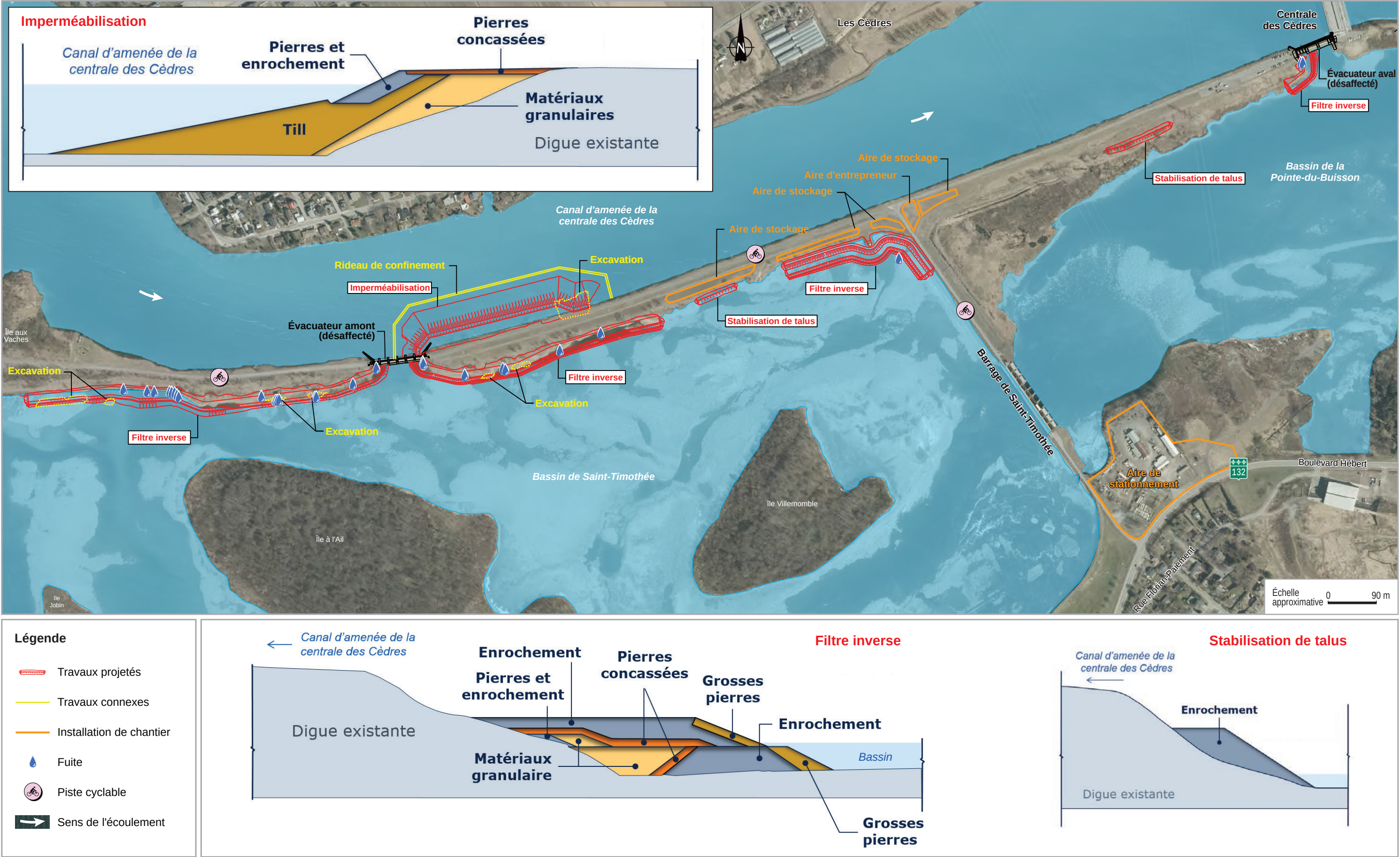
Figure 3 Les travaux projetés le long de la digue de la centrale des Cèdres
