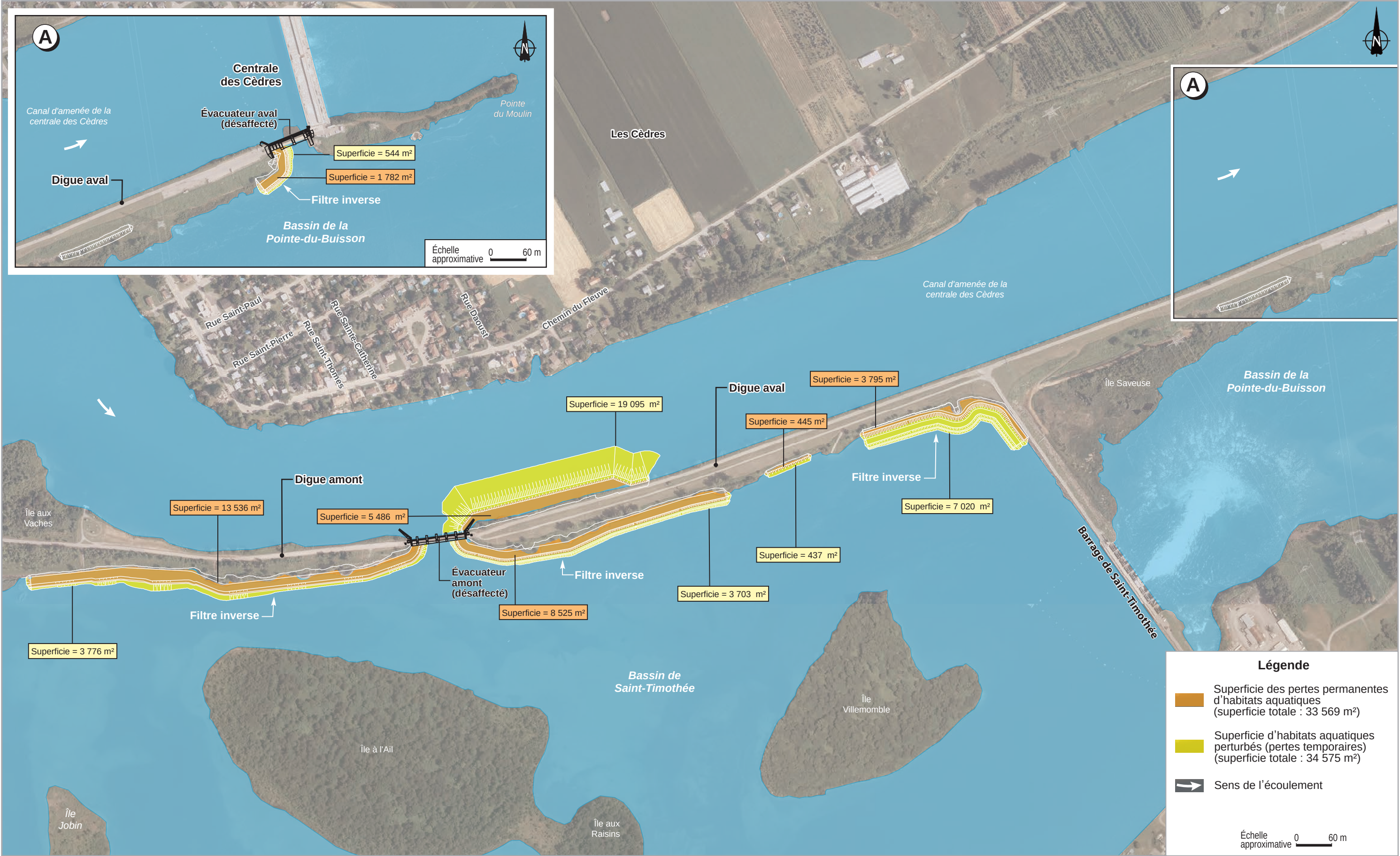
Figure 4 Les superficies des pertes et des perturbations d'habitats aquatiques
