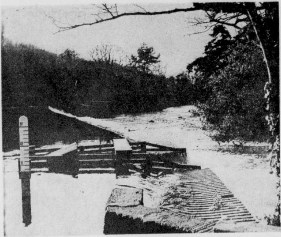
Ce barrage sur la rivière Leven, dans le nord-ouest de l'Angleterre, contient un tunnel de comptage de poissons. L'équipement installé sur ces lieux donne non seulement des renseignements inappréciables sur la vie des poissons de rivière, mais il permet aussi de montrer comment on peut satisfaire à tous les besoins privés et industriels sans pour autant menacer la vie des poissons.
