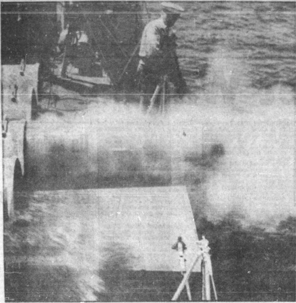
LA TORPILLE-ROBOT — La Marine canadienne, qui entrevoit la possibilité d'armer ses contre-torpilleurs de projectiles téléguidés, possède déjà quelques spécimens de cet engin: la torpille-robot. La photo montre le navire côtier d'escorte Sault-Ste-Marie en train de lancer une torpille-robot au cours d'un exercice. (Photo de la "PC")
