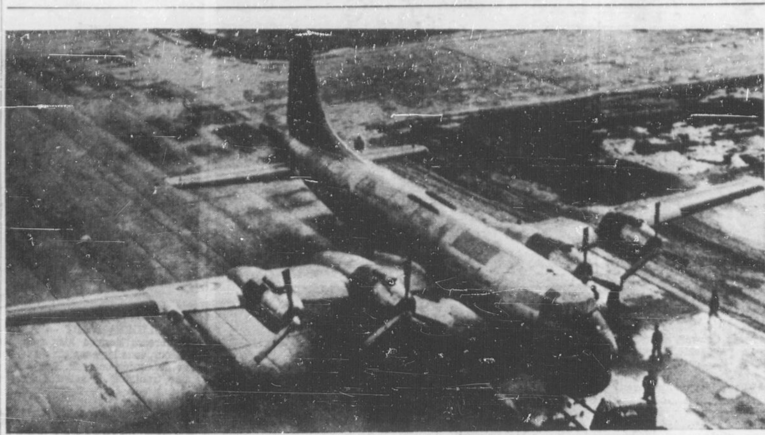
NOUVEAU CHASSEUR ANTISOU-MARIN — Cette photo nous montre le gigantesque chasseur antisou-marin CL-28 de la compagnie Canadair sur la piste d'envol, en route vers le hangar de préparation au vol, immédiatement après avoir quitté la ligne d'assemblage de cette usine de Montréal. Ce CL-28 est le premier d'une série qui seront fabriqués pour le commandement maritime du CARC. C'est le plus gros avion de sa catégorie jamais fabriqué au Canada. (Téléphoto "Le Droit" — de la PC)
