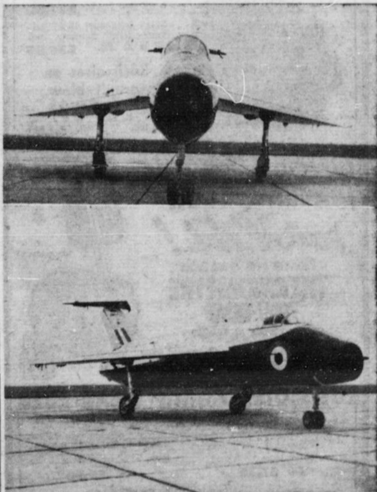
NOUVEL APPAREIL DE RECHERCHES. — Les Britanniques continuent leurs recherches dans le domaine de l'aéronautique. Ci-haut, un nouveau modèle qui servira à faire des expériences en plein vol, a été récemment piloté par le chef des épreuves Tom Brook Smith, de la firme Short. L'avion est propulsé par un seul moteur Rolls-Royce "turbo-jet". C'est le seul appareil anglais dont les ailes soient si retirées à l'arrière, afin de diminuer la résistance de l'air sur les bords d'attaque. Ceux-ci, en relation avec le fuselage, sont fixés à un angle de 50 degrés et sont mobiles, permettant ainsi un plus grand nombre d'expériences.
