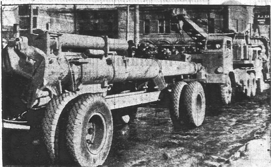
Ce canon géant est un howitzer 240 millimètres. Il a été photographié quittant une usine de Milwaukee pour se rendre à Aberdeen, Maryland, où il doit subir des essais. Il appert que c'est le plus gros howitzer entièrement mobile qui ait été construit.
