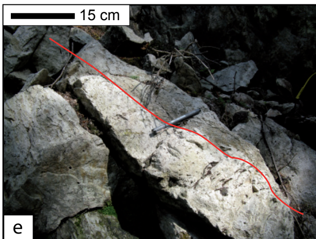
FIGURE 2 - Photos d'affleurement de certaines unités de la Formation d'Hébécourt : a ) basalte coussiné de l'unité Aht1 montrant une jonction triple avec de la hyaloclastite interstitielle; b ) faciès massif de la rhyolite de l'unité Aht4a, avec phénocristaux de quartz et de plagioclase de 1-2 mm, et recoupé par de minces veinules de séricite; c ) faciès bréchiqye de la rhyolite aphyrique de l'unité Aht4b; d ) même faciès, illustrant un fragment plus vésiculaire (à gauche); e ) faciès massif de la rhyolite aphyrique (unité Aht4b) montrant le contact entre deux lobes (ligne rouge); f ) coussin rencontré dans l'unité d'andésite basaltique Aht5 montrant une augmentation de la concentration d'amygdales et de varioles vers sa bordure.
