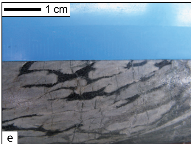
FIGURE 3 - Photos de carottes de forage, illustrant certaines unités volcaniques et certains niveaux laminés riches en sulfures de la Formation d'Hébécourt : a ) premier niveau laminé riche en sulfures contenant un sédiment tuffacé laminé, interlité avec des couches riches en pyrite (HEB-04, 374,4 m); b ) brèche de coussins dans l'andésite basaltique de l'unité Aht5 montrant des fragments de forme irrégulière, faisant jusqu'à 10 cm de large, entourés de hyaloclastite présentant par endroits une texture de mosaïque (HEB-02, 263,1 m); c ) jonction triple entre des coussins dans l'andésite basaltique de l'unité Aht5 (HEB 04, 71,4 m). La hyaloclastite remplissant l'espace interstitiel est imprégnée de sulfures; d ) tuf à lapillis de l'unité Aht6 (rhyolite), montrant un domaine moins altéré à droite, entouré de roche silicifiée à gauche (HEB-02, 193,7 m); e ) rhyolite massive de l'unité Aht6 montrant des sphéroïdes aplatis par la déformation (HEB-02, 168,8 m); et f ) second niveau laminé riche en sulfures contenant de l'argilite et de la pyrite (HEB-02, 140,2 m). Une partie de la pyrite est associée à une veinule de quartz.
