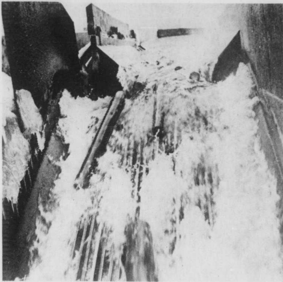
Le bois arrive à l'usine de Tembec en billes ou en copeaux. Les billes descendent la rivière par flottage, jusqu'aux stations de stockage et postes de triage. Elles sont ensuite acheminées vers quatre tambours-écorceurs Ingersoll-Rand, qui les écorcent, avant de passer dans deux puissantes déchiqueteuses, qui les transforment en copeaux ouvrables.
