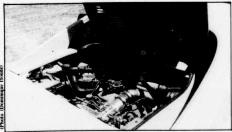
Le 2 litres turbocompressé à 16 soupapes de la MR2 est brillant à haut régime. mais discret sous la barre des 3500 tr / mn.
