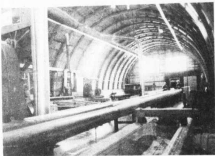
Vue du convoyeur qui conduit le bois à la scie double pour régulariser.
