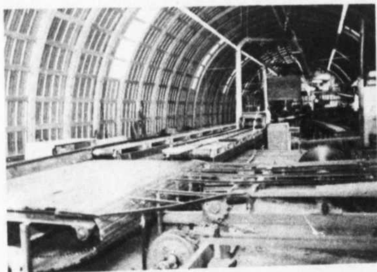
Vue en partie de la scie double mais aussi vue générale du moulin.
