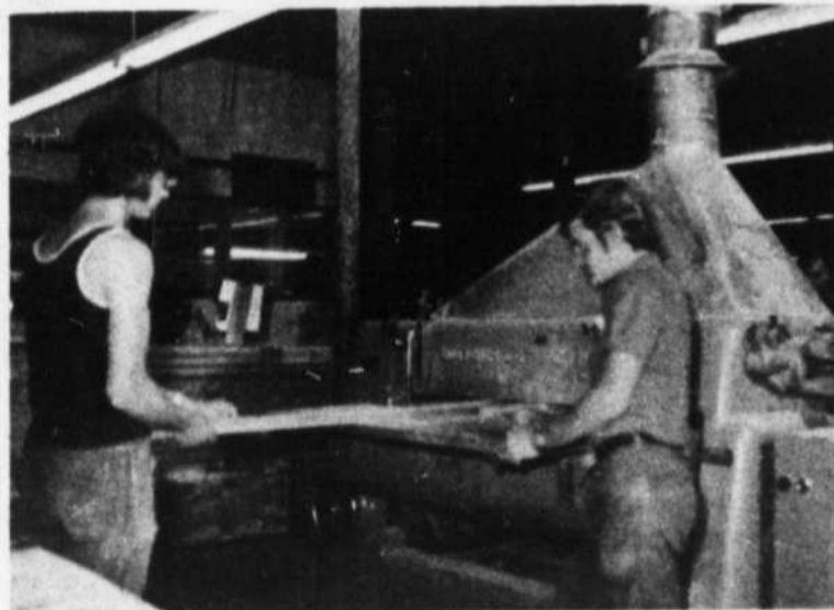
Réjean Croteau, contremaître du département de débitage et machinage explique une nouvelle opération à M. Claude Houle opérateur d'une sableuse.
