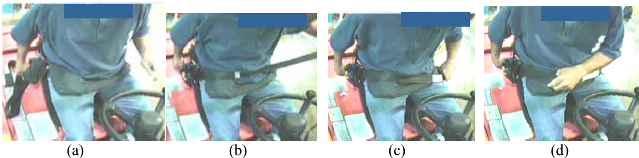
Figure 16. Phases typiques du bouclage avec le rétracteur manuel – avec ajustement.
