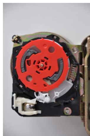
Figure 5. Vue intérieure latérale d'un rétracteur ELR à bille.
