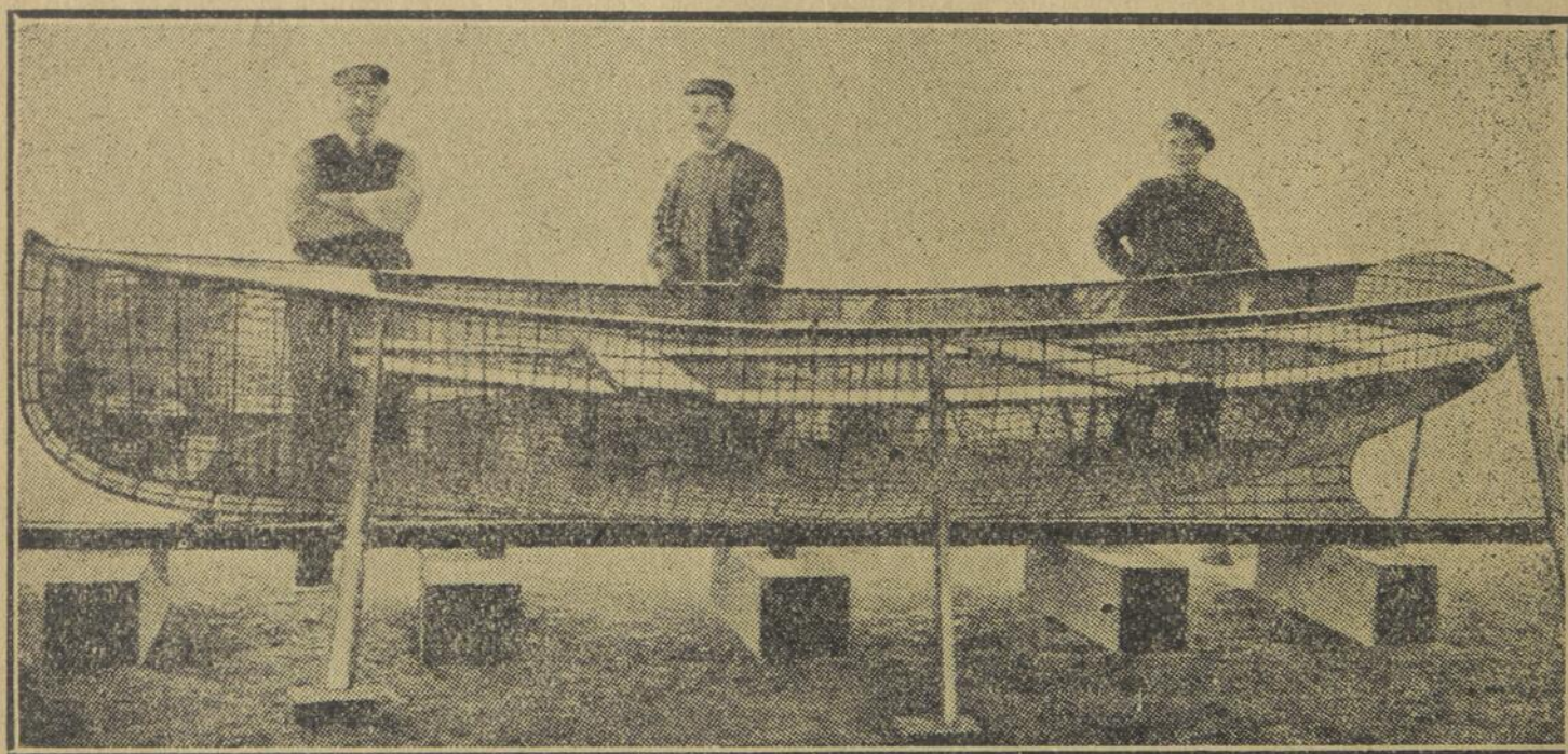
Armature de canot automobile en ciment armé.
