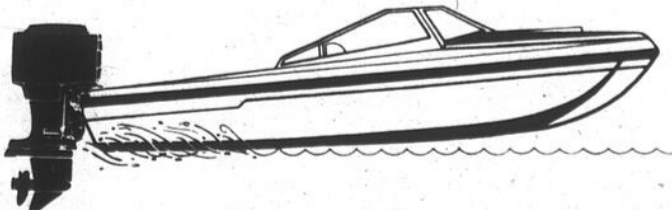
Le fond du bateau est approximativement à 3° de la surface de l'eau. Position idéale de croisière, le bateau et le hors-bord sont dans un angle parfait. Vitesse, économie, sécurité et confort en résultent de vous dire les distributeurs des hors-bords Mercury.
