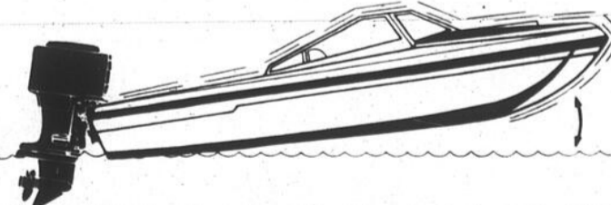
La proue est trop haute; le hors bord trop incliné vers l'extérieur. L'embarcation saute en surface comme un dauphin, la flèche de l'avant indiquant le mouvement de haut en bas.
