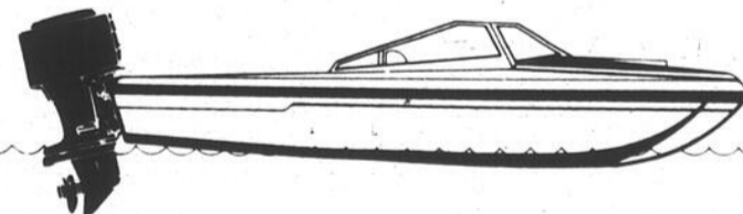
La proue est trop basse; le hors bord trop incliné vers l'intérieur. L'embarcation semble vouloir plonger et faire de grosses vagues.
